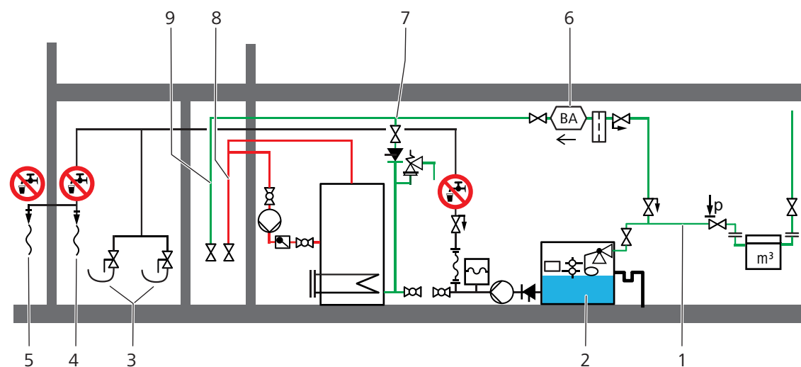
Fig. 8: Exemple d'une installation dans une exploitation d'élevage. Remarque: Les abreuvoirs sont dans ce cas sécurisés via la station de séparation et de sécurité.
