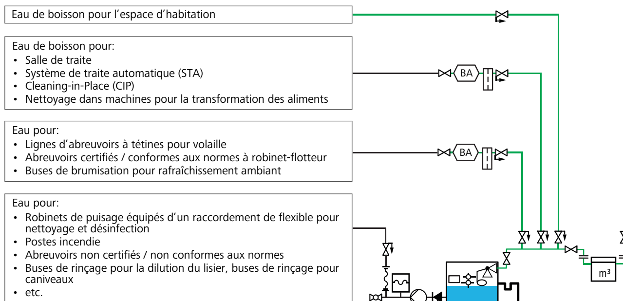
Fig. 7: Schéma de principe dispositifs de protection pour divers usages (adaptation libre notice technique SVGW W10030:2025, chapitre 4.1)
