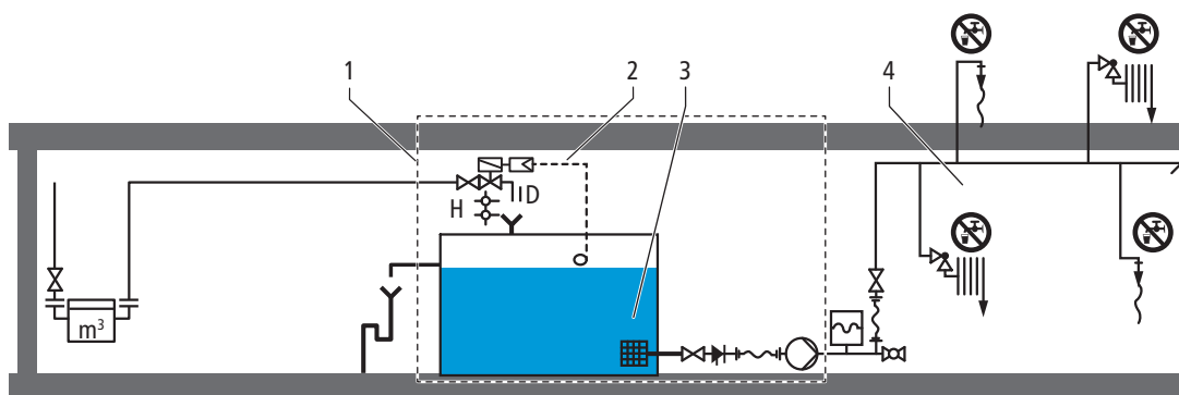
Fig. 12: Protection contre les retours d'eau dans des installations d'épuration des eaux, fig. 5 de la notice technique W10035:2023, chapitre 6
