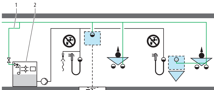
Fig. 11: Raccordement d'une douchette pour WC avec station de séparation et de sécurité AB, fig. 1 de la notice technique 10032:2019, chapitre 3.3
