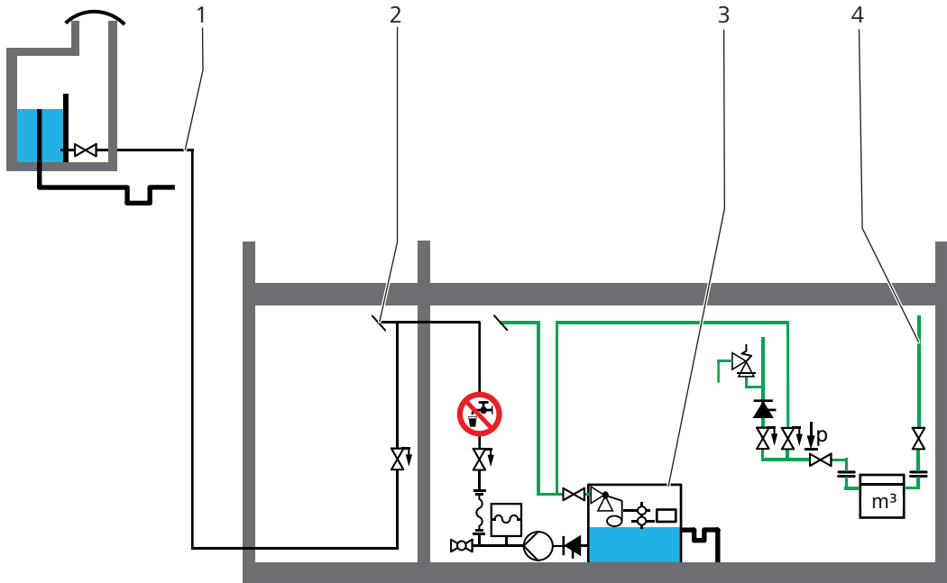
Fig. 9: Séparation des réseaux privé et public d'eau de boisson avec surverse AB, fig. 19 de la notice technique 10030:2025, chapitre 10.3
