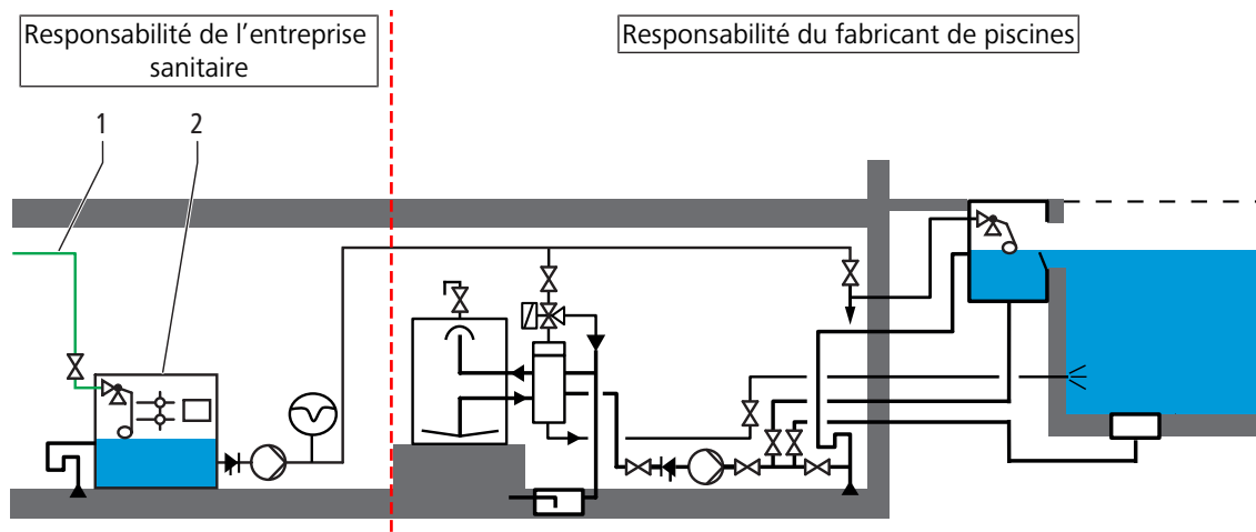
Fig. 10: Réalimentation d'une piscine avec station de séparation et de sécurité AB, fig. 7 de la notice technique 10009:2017, chapitre 6
