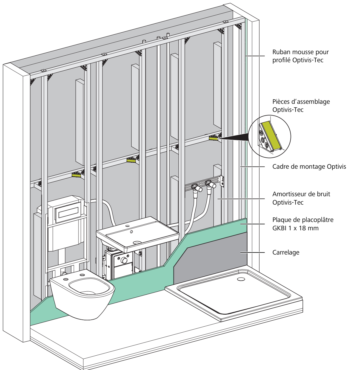
Fig. 15: Cadre de montage Optivis équipé de sanitaires
