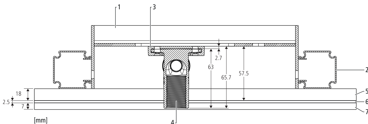
Fig. 6: Module de support robinetterie Optivis-Tec, parement simple
