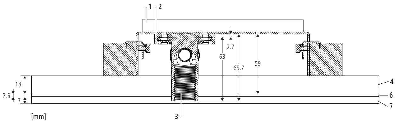
Fig. 10: Module GIS Optiflex-Profix, parement simple 18 mm
