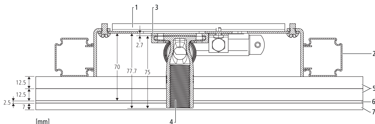
Fig. 9: Module lavabo Optivis-Tec, parement double
