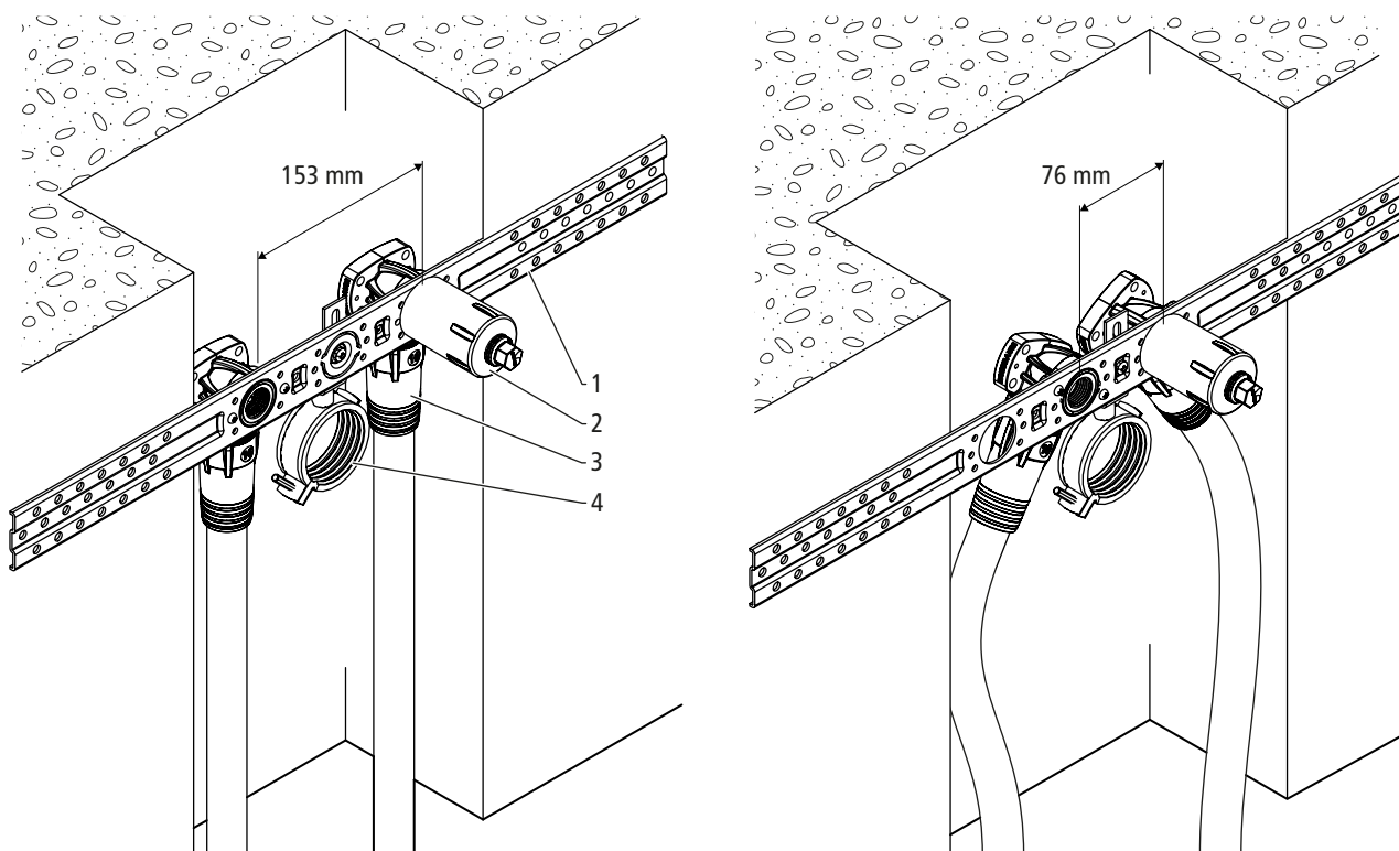
Fig. 1: Boîtes écartées de 153 et 76 mm avec gabarit de montage 85056
