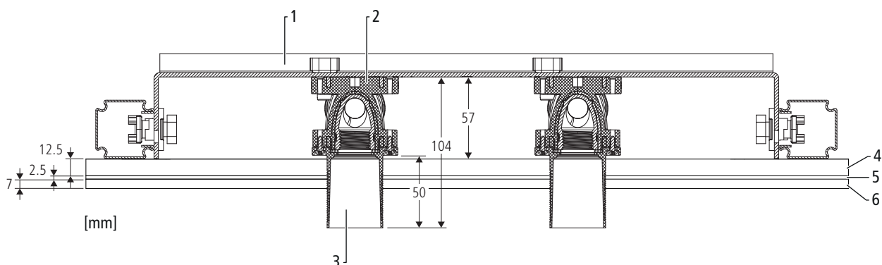
Fig. 12: Module Optiflex-Optivis, parement simple 84214/85214
