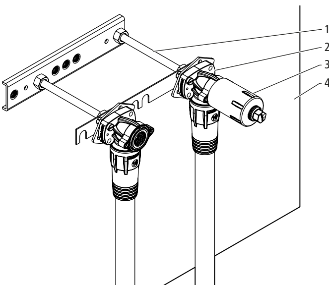
Fig. 5: Cadre de montage
