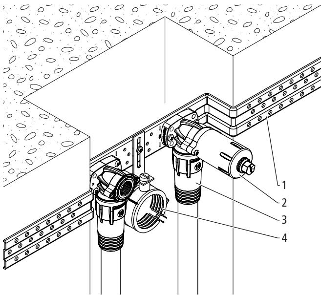
Fig. 2: Montage dans l'évidement dans un mur
