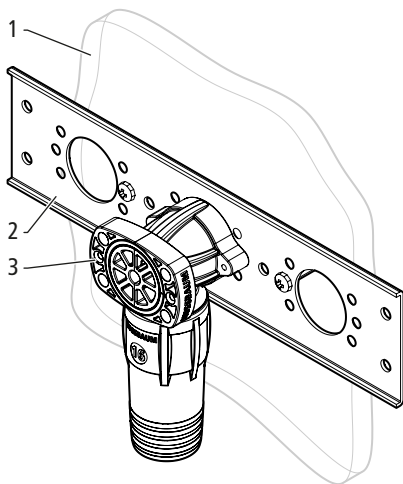
Fig. 4: Montage sur mur en bois
