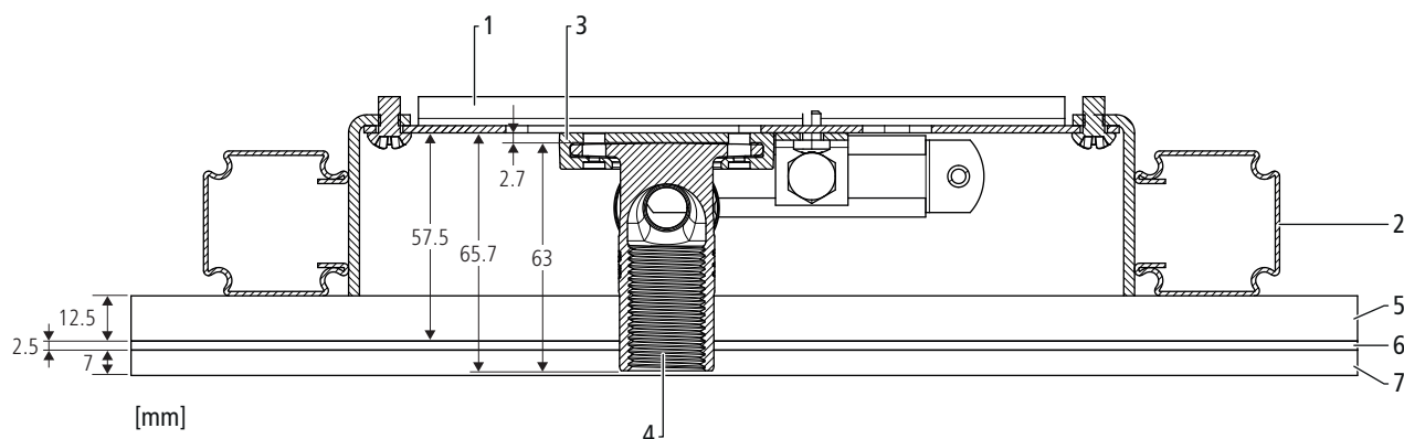
Fig. 8: Module lavabo Optivis-Tec, parement simple
