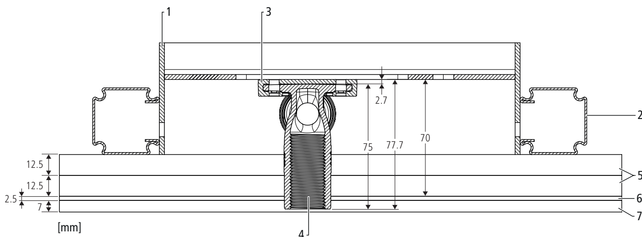
Fig. 7: Module de support robinetterie Optivis-Tec, parement double
