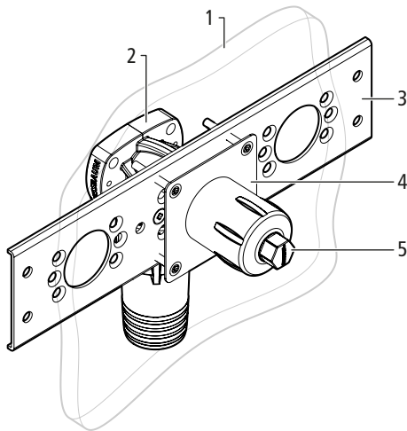
Fig. 3: Montage sur mur en plâtre
