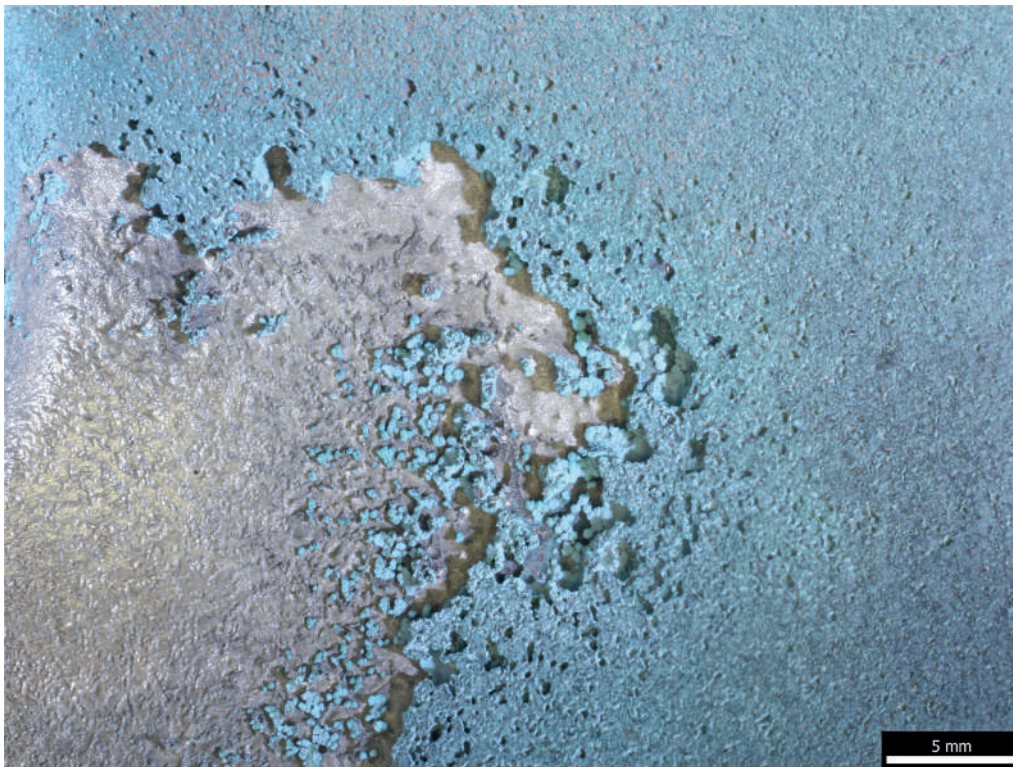
Fig. 25: Vue détaillée des dommages
