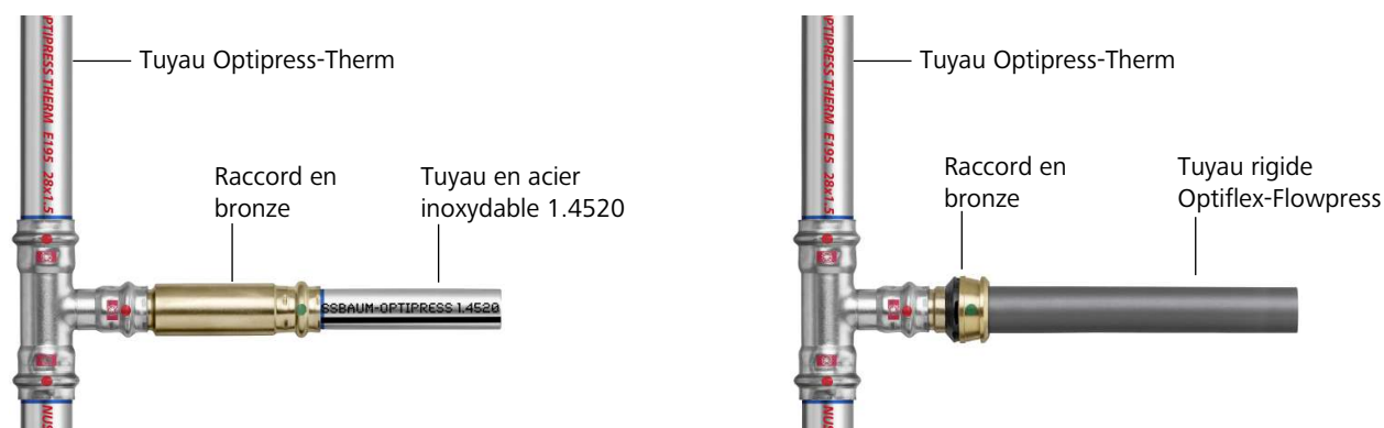
Fig. 54: Installations mixtes admissibles d'Optipress-Therm sur Optipress-Aquaplast et Optiflex-Flowpress
