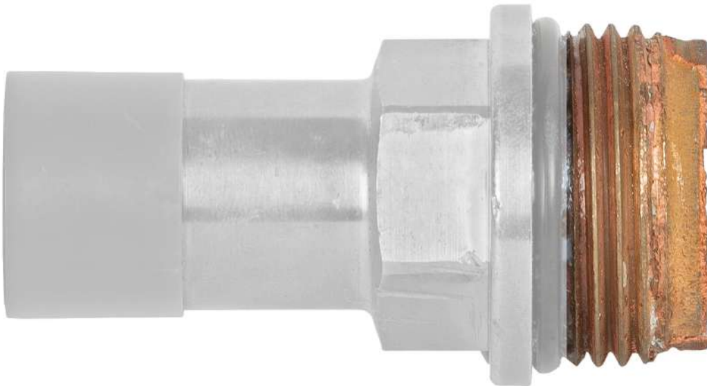
Fig. 27: Dommages par dézincification du filetage d'une tête de robinet
