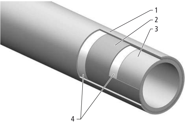
Fig. 58: Tuyau Optiflex-Flowpress rigide
