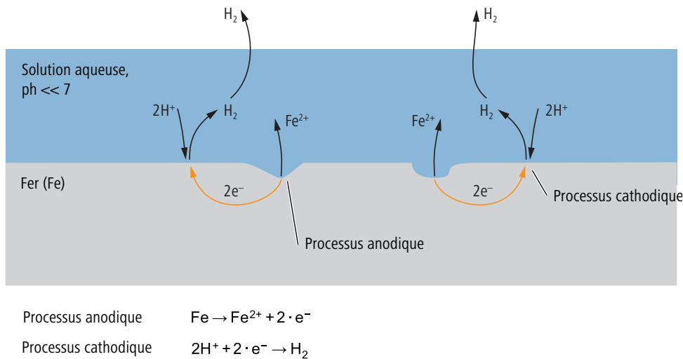
Fig. 7: Corrosion du fer par hydrogène dans une solution aqueuse fortement acide
