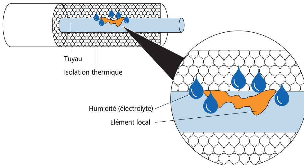
Fig. 44: Corrosion sous une isolation thermique
