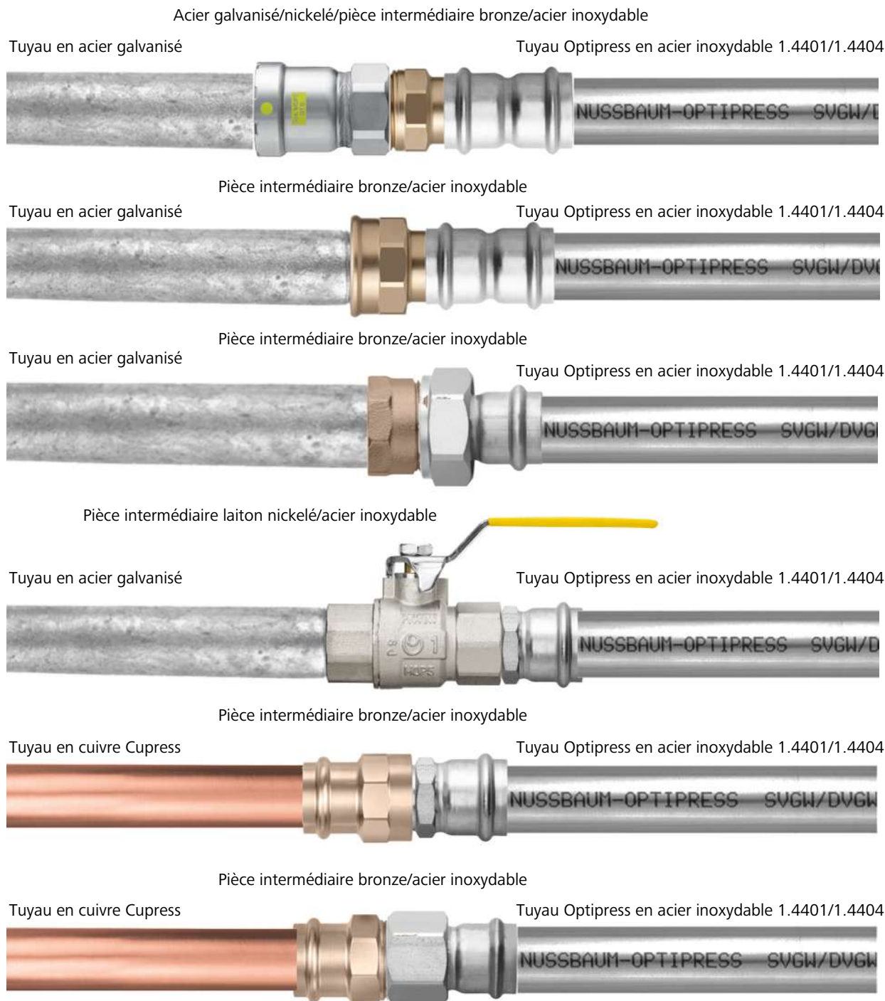
Fig. 56: Installations mixtes admissibles avec Optipress-Gaz
