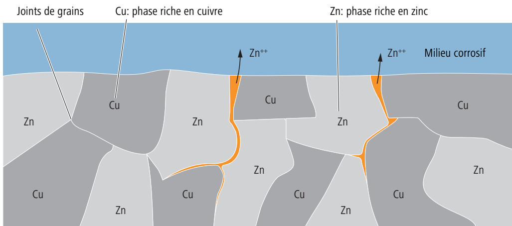
Fig. 28: Corrosion intercrystalline (schéma: Bickle et autres, Technique d'installation)
