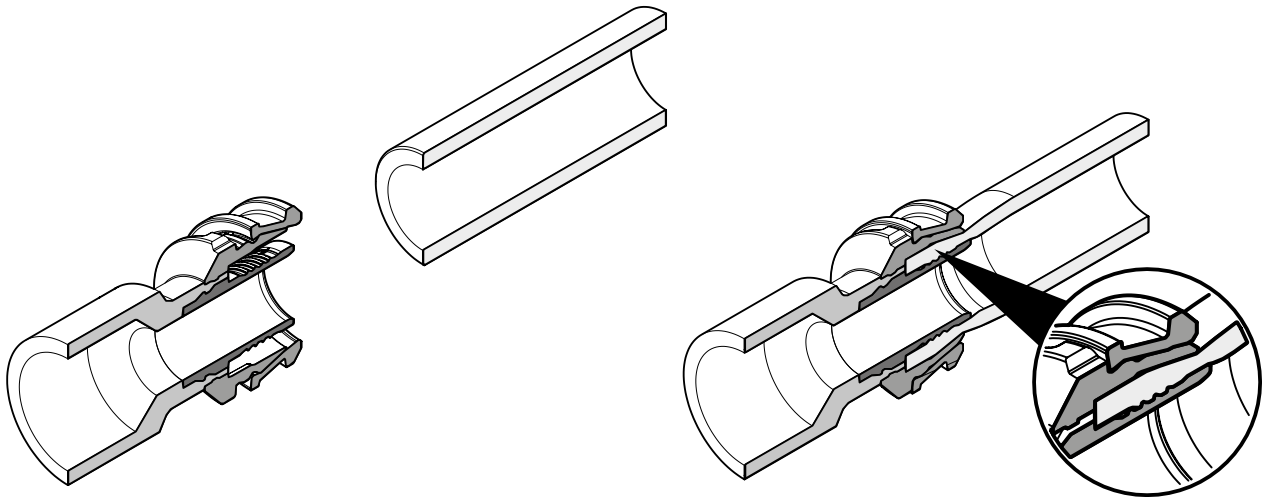
Abb. 6: Optiflex-Flowpress-Verbindung (offen/verpresst)
