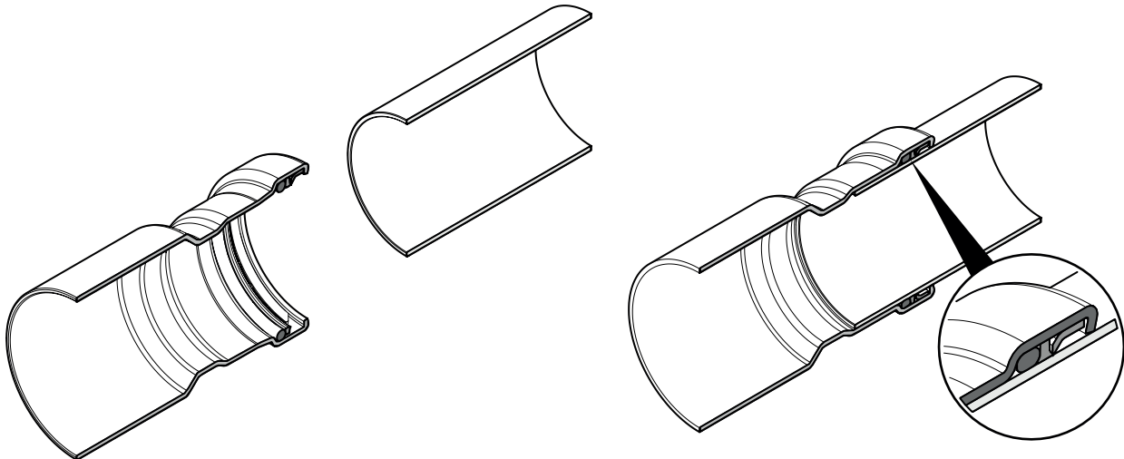
Abb. 3: Optipress-XL-Verbindung (offen/verpresst)
