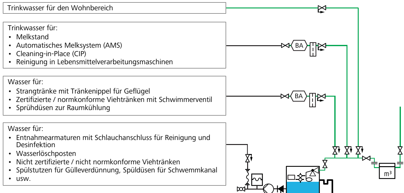
Abb. 7: Prinzipschema Sicherheitseinrichtungen für unterschiedliche Verwendungszwecke (frei nach SVGW-Merkblatt W10030:2025, Kapitel 4.1)
