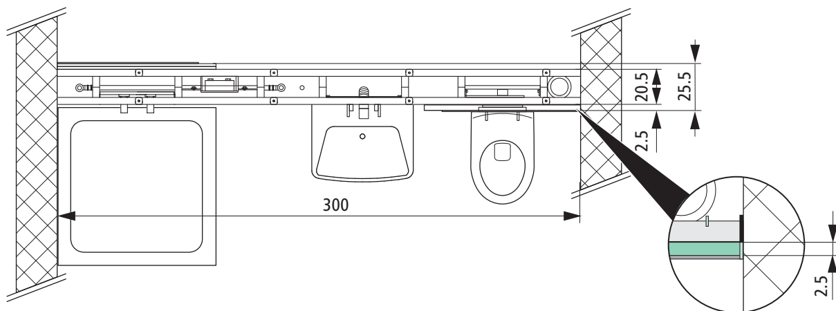
Abb. 21: Grundriss
