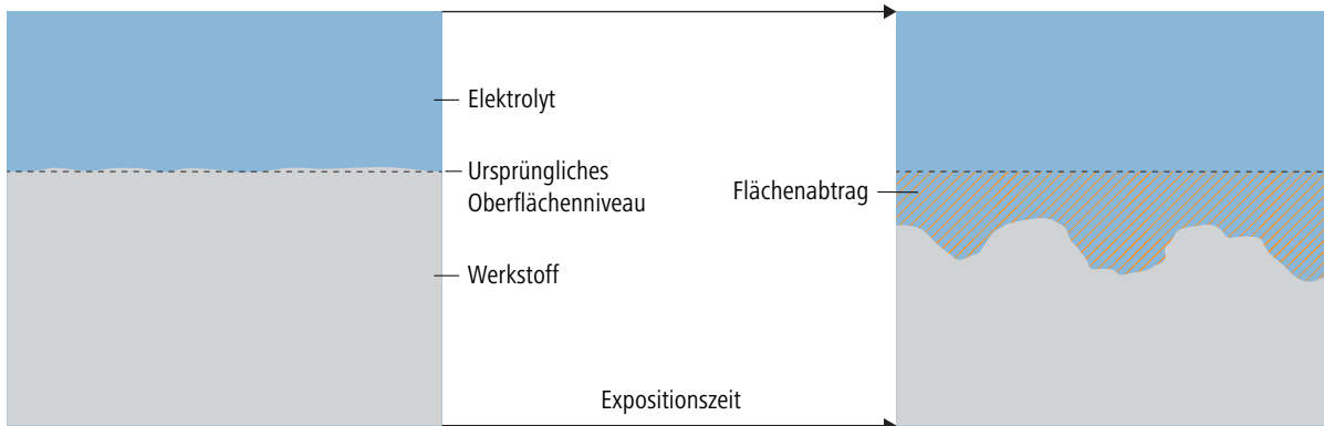
Abb. 12: Flächenkorrosion
