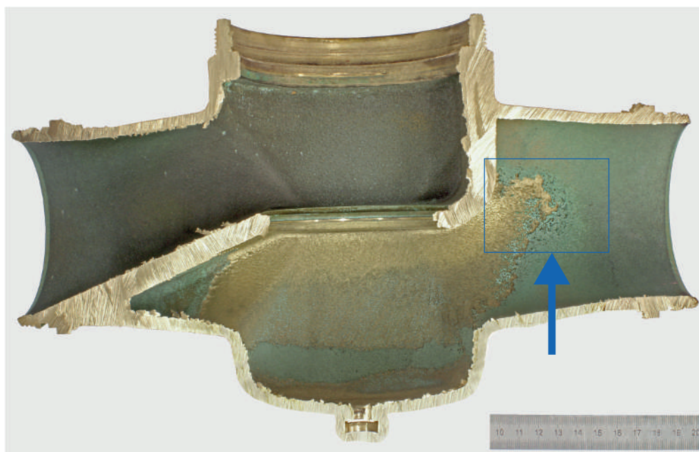
Abb. 24: Schadenbild einer Mischform von Erosions- und Kavitationskorrosion
