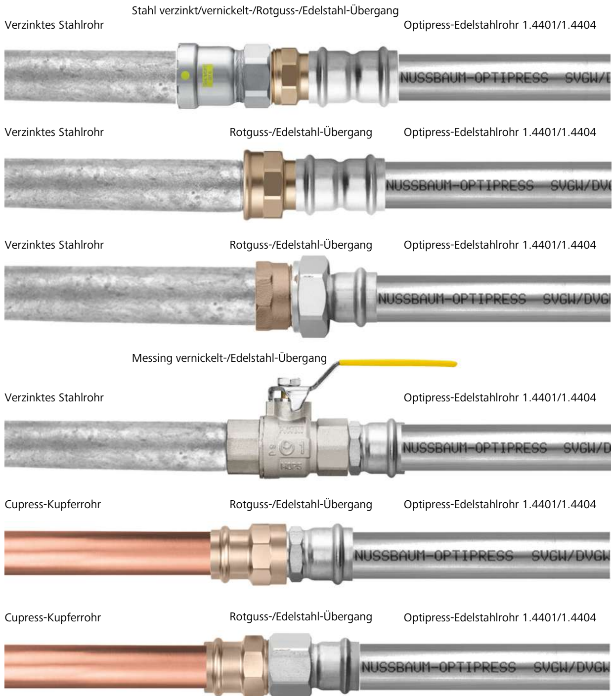
Abb. 56: Zulässige Mischinstallationen mit Optipress-Gaz
