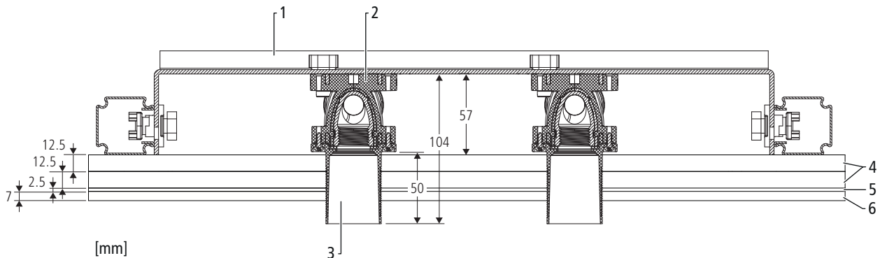
Abb. 11: Optivis-Tec-Modul 2-fach beplankt 84214/85214
