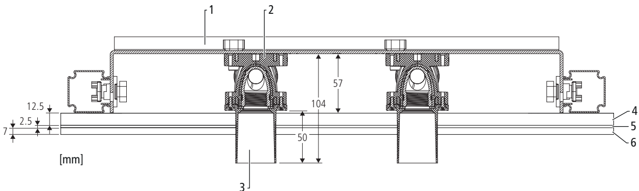
Abb. 10: Optivis-Tec-Modul 1-fach beplankt 84214/85214
