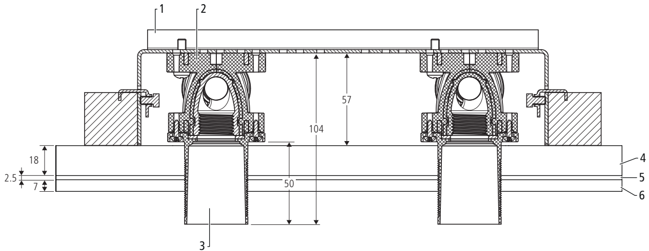
Abb. 9: Optiflex-GIS-Modul 1-fach beplankt 18 mm 85121/84221
