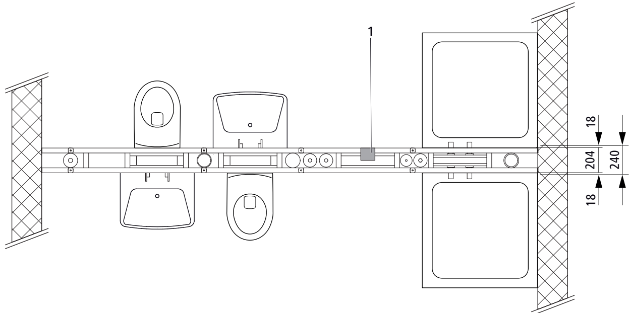
Abb. 17: Optivis-Tec-Trennwand 240 mm beidseitig belegt
