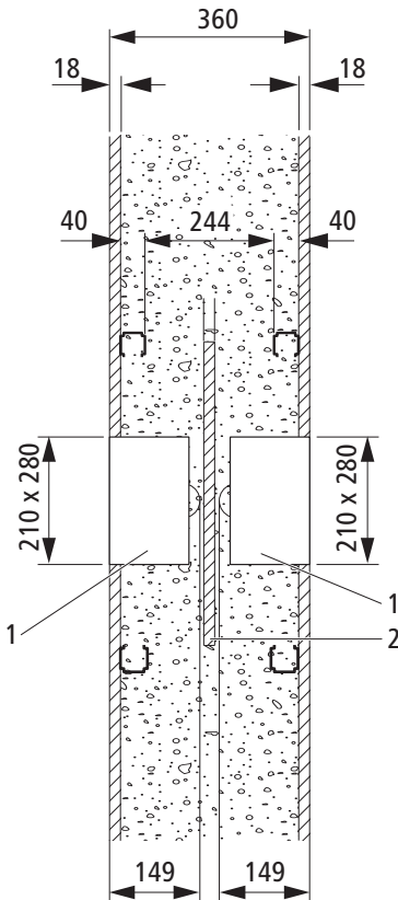
Abb. 11: Beidseitiger Einbau in Optimis-Tec-Trennwand 360 mm
