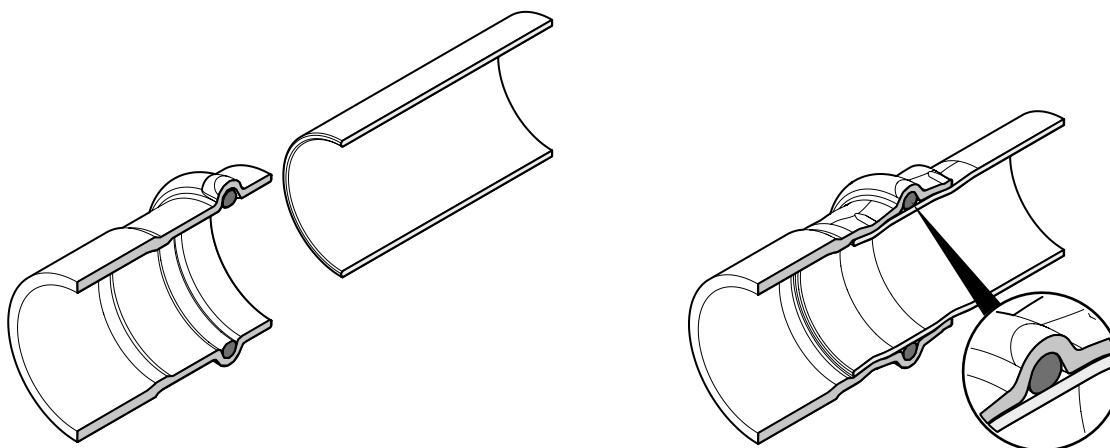
Fig. 1: Collegamento Optipress (aperto/pressato)
