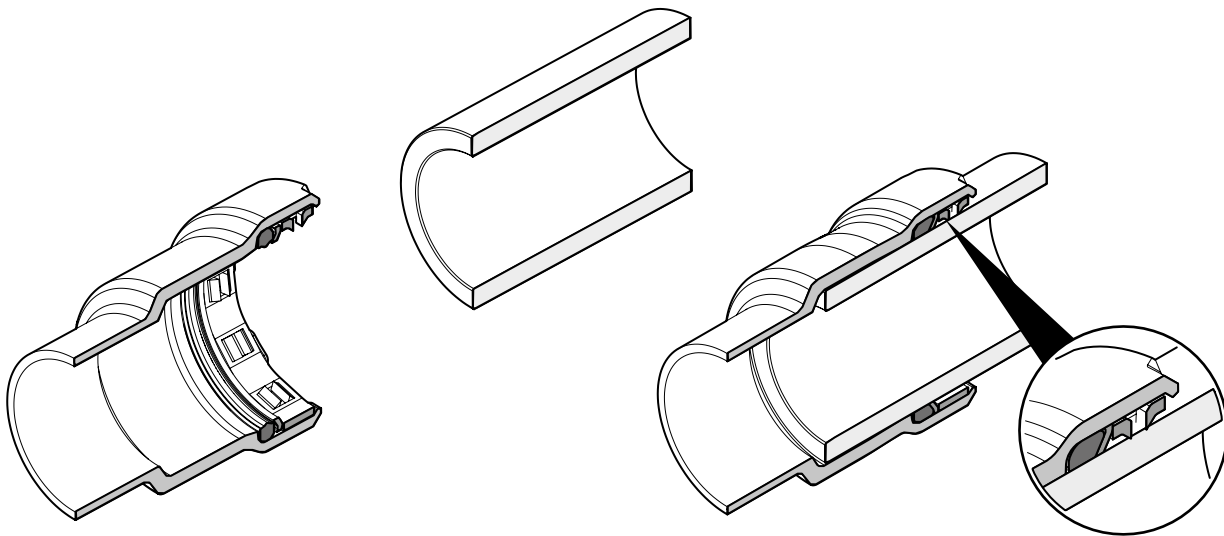
Fig. 5: Collegamento Optifitt-Press (aperto/pressato)
