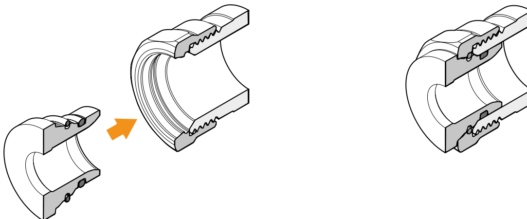
Fig. 11: Collegamento a innesto (aperto/inserito)
