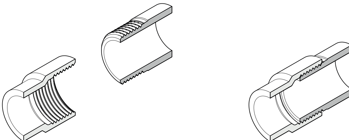
Fig. 12: Collegamento filettato per tubi a norma ISO 7-1/EN 10226 (non avvitato / avvitato)
