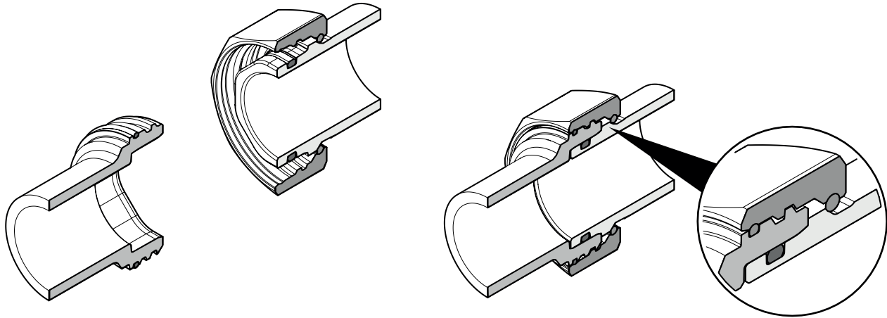
Fig. 10: Accoppiamento rapido (aperto/chiuso)
