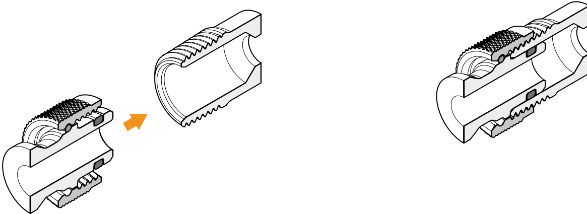
Fig. 17: Adattatore MF (aperto/chiuso)
