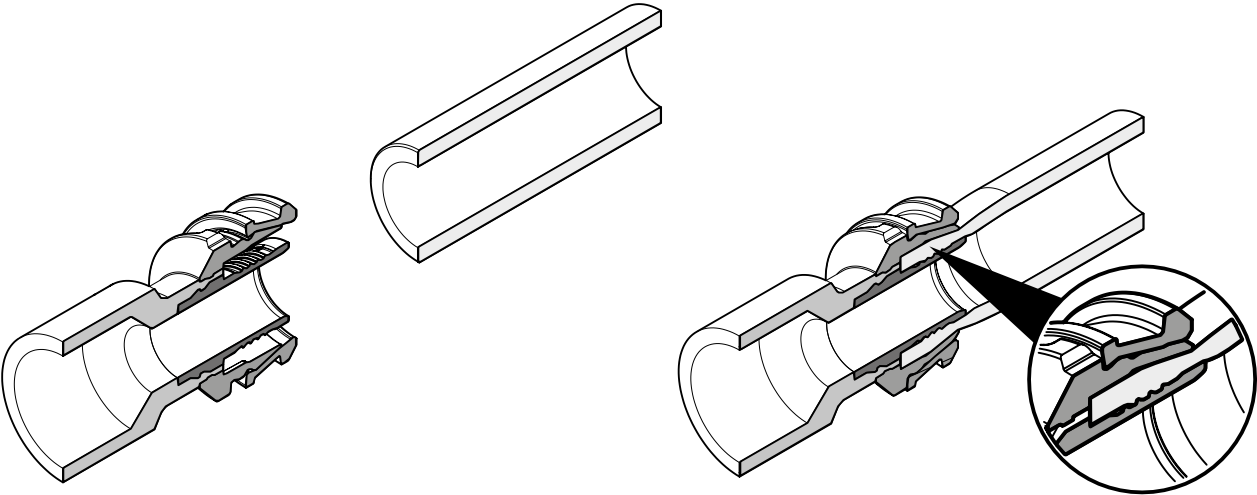
Fig. 6: Collegamento Optiflex-Flowpress (aperto/pressato)
