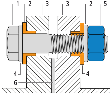
Fig. 16: Collegamento a flangia avvitato con bussole a colletto
