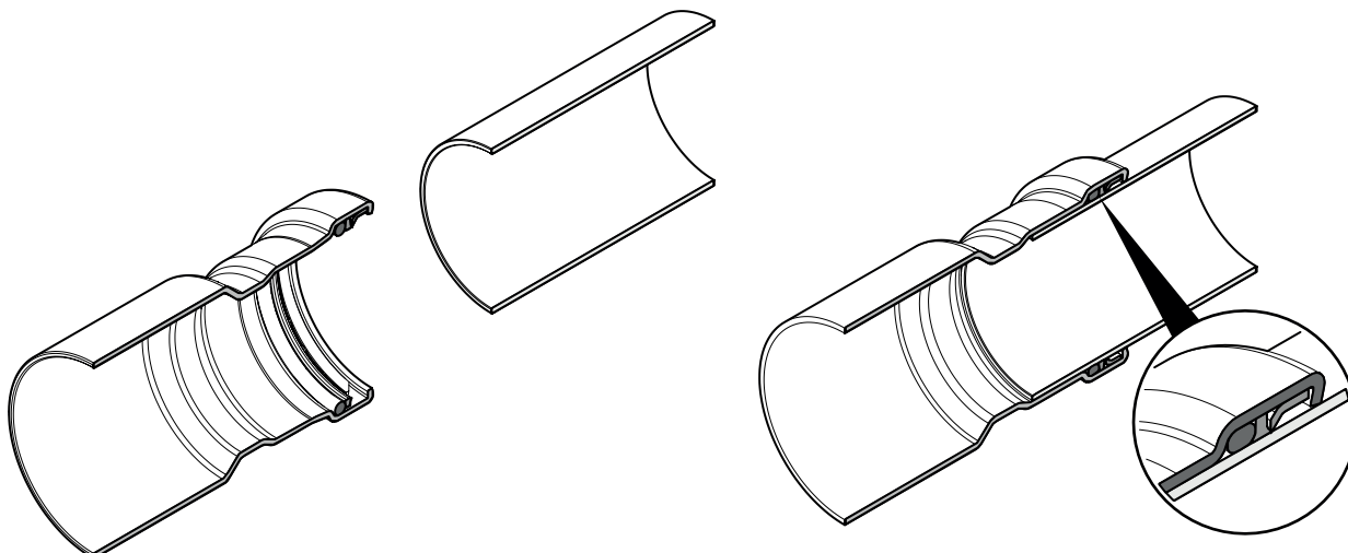
Fig. 3: Collegamento Optipress XL (aperto/pressato)
