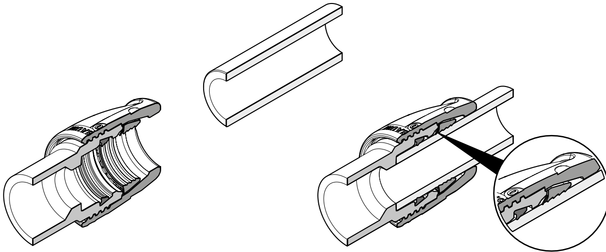
Fig. 8: Collegamento Optiflex-Profix (aperto/inserito)
