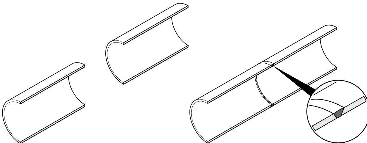
Fig. 18: Collegamento a saldare (aperto/saldato)
