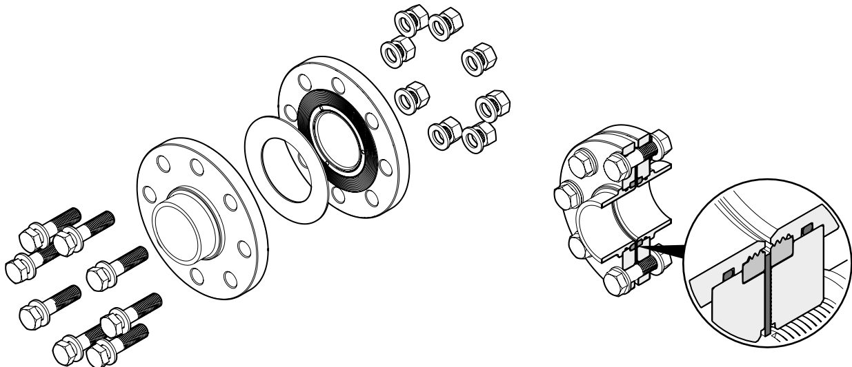
Fig. 15: Collegamento a flangia ruotabile (non avvitato / avvitato)
