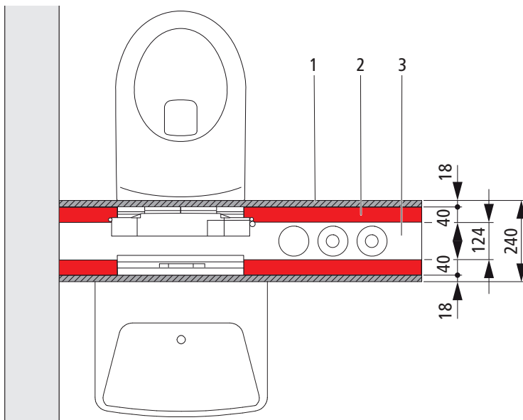
Fig. 18: Vista dettagliata sezione parete divisoria 240 mm
