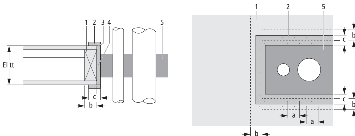
Fig. 16: Installazione Optimis-Tec in costruzione in legno con colletto RF1
