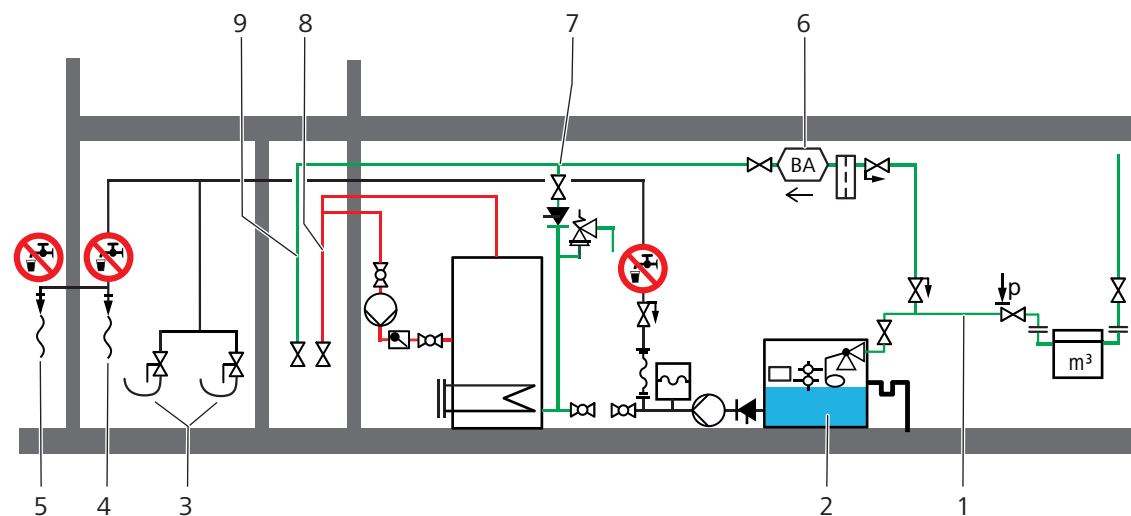
Fig. 8: Esempio di impianto in azienda zootecnica. Nota: In questo caso, gli abbeveratoi sono protetti tramite la stazione di separazione e sicurezza.
