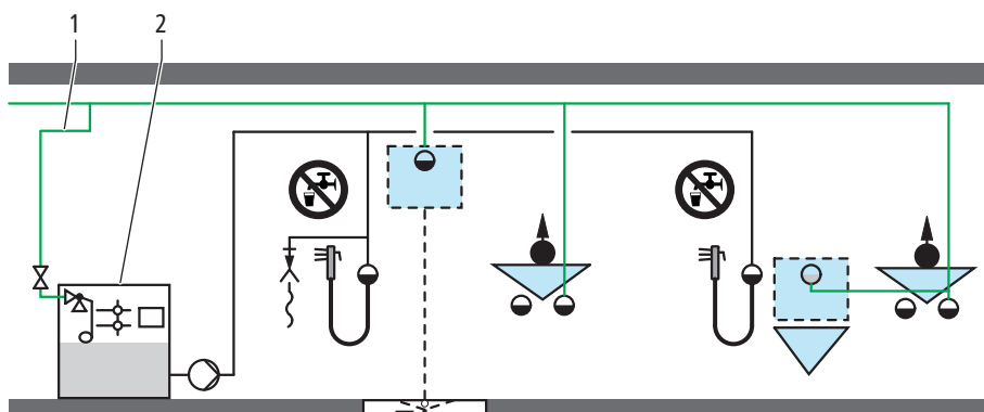
Fig. 11: Collegamento di una doccetta per WC con stazione di separazione e sicurezza AB, fig. 1 della nota tecnica W10032:2019, capitolo 3.3.
