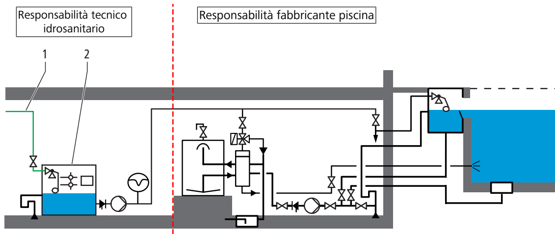
Fig. 10: Riempimento di piscine con stazione di separazione e sicurezza AB, fig. 7 della nota tecnica W10009:2017, capitolo 6.
