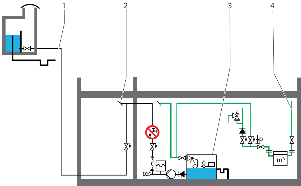
Fig. 9: Separazione dell'approvvigionamento idrico privato e pubblico mediante scarico libero AB, fig. 19 della nota tecnica W10030:2025, cap. 10.3.
