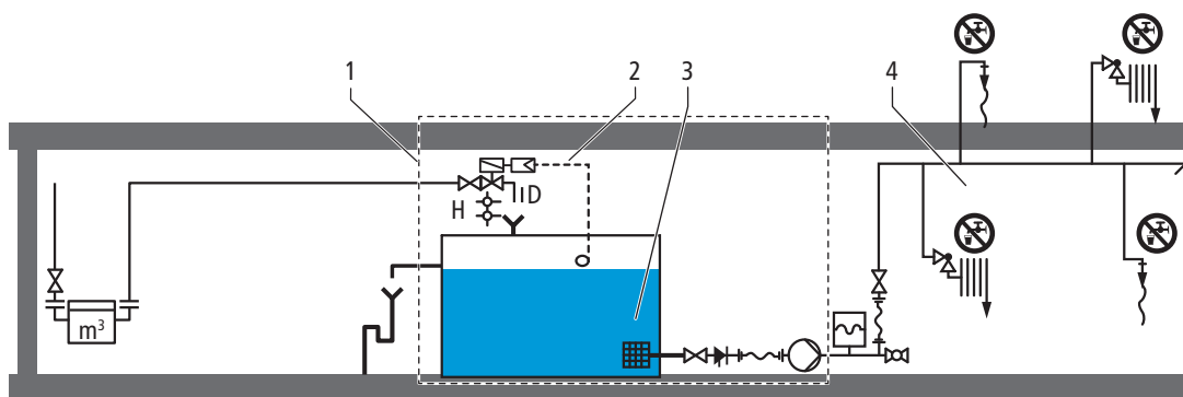
Fig. 12: Impedimento del reflusso in impianti di depurazione delle acque di scarico, fig. 5 della nota tecnica W10035:2023, capitolo 6
