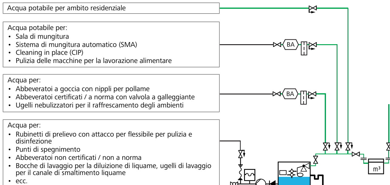
Fig. 7: Schema di principio dispositivi di protezione per diversi scopi (liberi secondo la nota tecnica W10030:2025 della SVGW, cap. 4.1)
