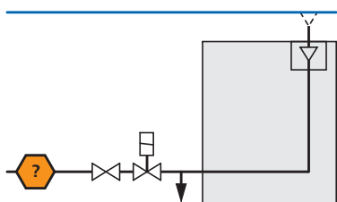
Fig. 2: Esempio di p > atm : irrigazione del sottosuolo.
