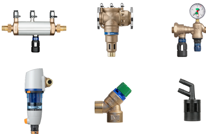
Fig. 5: Esempi di rubinetti con scarico libero sopra un elemento di drenaggio: disgiuntore di rete 15073 e 15087, gruppo per riempimento del riscaldamento 15092, Redfil 12100, valvola di sicurezza 13000, raccordo acqua di lavaggio 19098.
