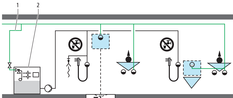
Fig. 9: Collegamento di una doccetta per WC con stazione di separazione e sicurezza AB, fig. 1 della nota tecnica W10032:2019, capitolo 3.3.
