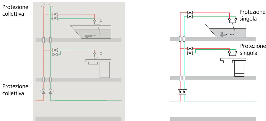
Fig. 3: Protezione collettiva obsoleta della condotta montante, non ammessa in Svizzera (a sinistra) vs. protezione individuale (a destra).
