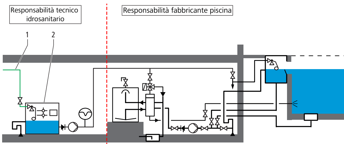
Fig. 8: Riempimento di piscine con stazione di separazione e sicurezza AB, fig. 7 della nota tecnica W10009:2017, capitolo 6.
