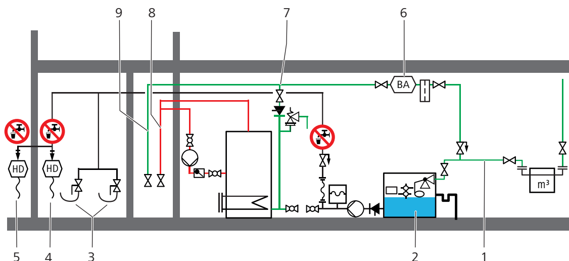
Fig. 6: Tipico impianto in azienda zootecnica secondo la nota tecnica W10030:2017 della SSIGA, capitoli 5 e 6.
