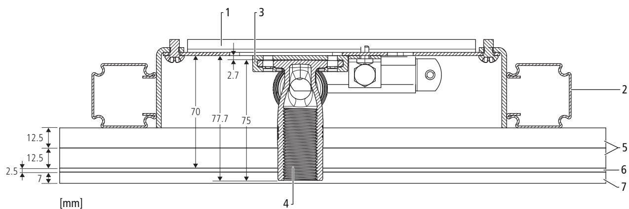
Fig. 12: Modulo per lavabo Optivis-Tec con rivestimento su due lati
