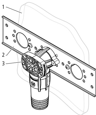
Fig. 7: Montaggio sulla parete in legno
