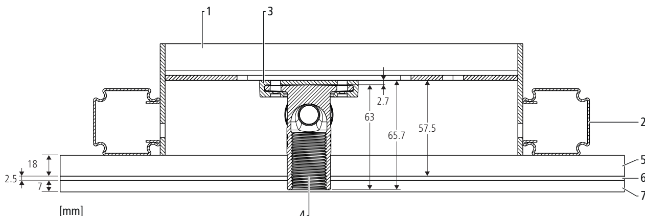
Fig. 9: Modulo porta-rubinetto Optivis-Tec con rivestimento su un lato
