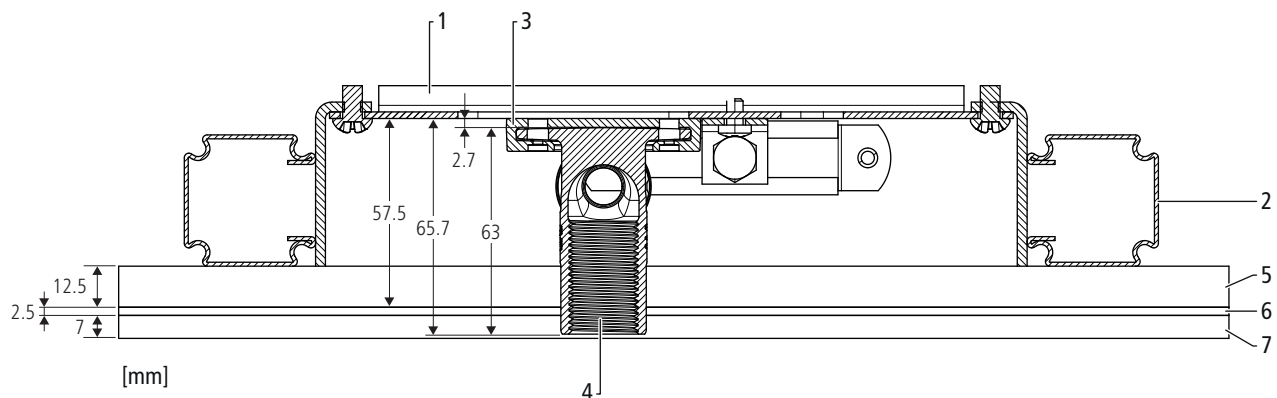
Fig. 11: Modulo per lavabo Optivis-Tec con rivestimento su un lato
