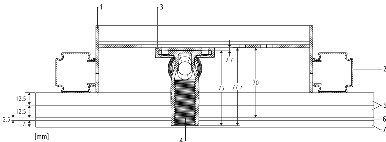
Fig. 10: Modulo porta-rubinetto Optivis-Tec con rivestimento su due lati
