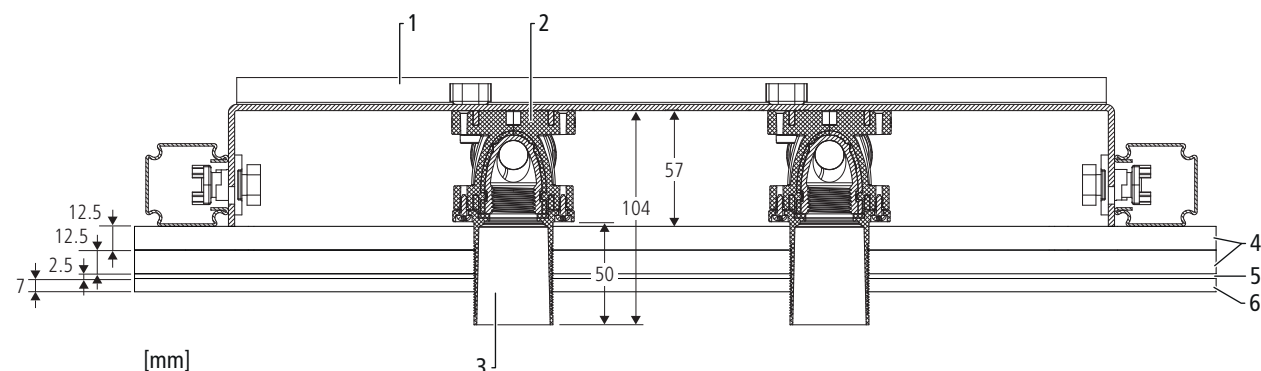
Fig. 16: Optivis-Tec-Modulo con rivestimento su due lati 84214/85214
