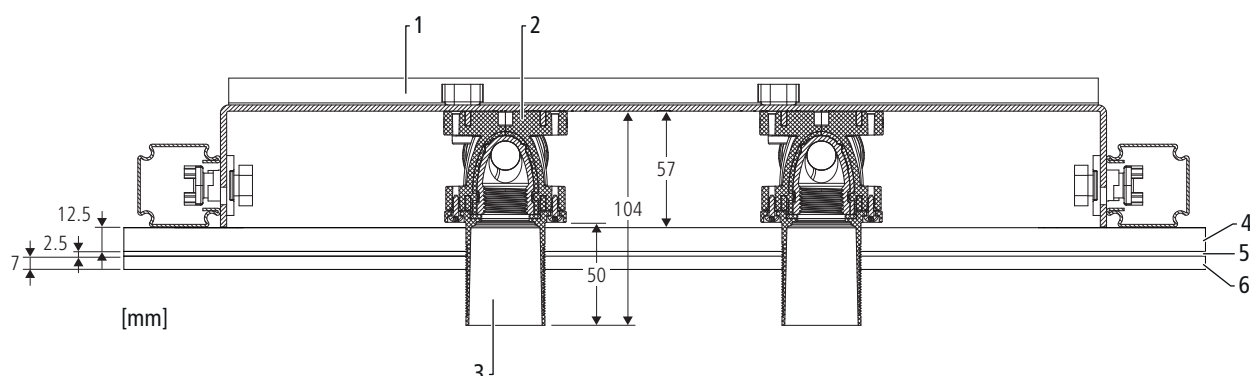
Fig. 15: Optivis-Tec-Modulo con rivestimento su un lato 84214/85214
