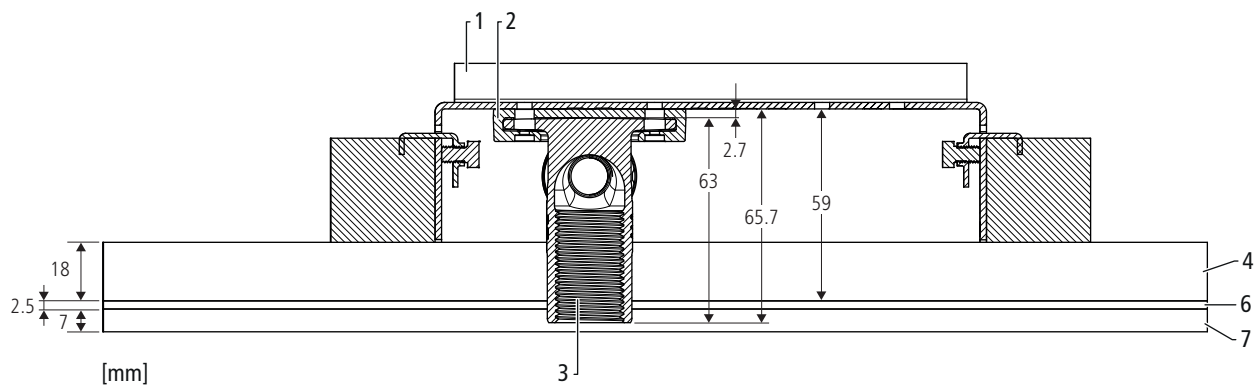
Fig. 10: Modulo Optiflex-Proflex GIS con rivestimento su un lato 18 mm
