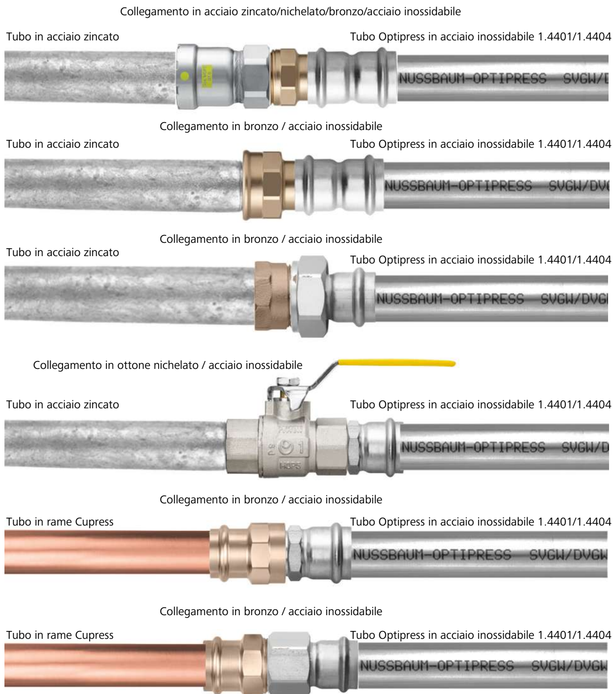
Fig. 56: Installazioni miste consentite con Optipress-Gaz
