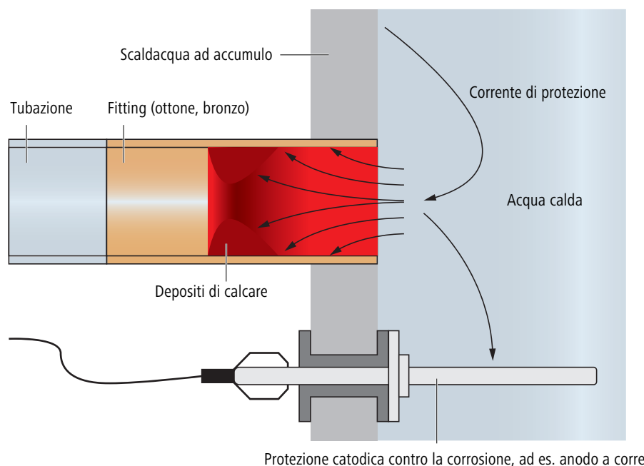
Fig. 37: Le correnti continue di impianti di protezione contro la corrosione possono provocare depositi di calcare nei fitting in ottone installati nell'area di collegamento di scaldacqua ad accumulo (immagine dal Promemoria suisse-tec W10019 «Ablagerung auf Messingfittings in Warmwasserkreisläufen»).
