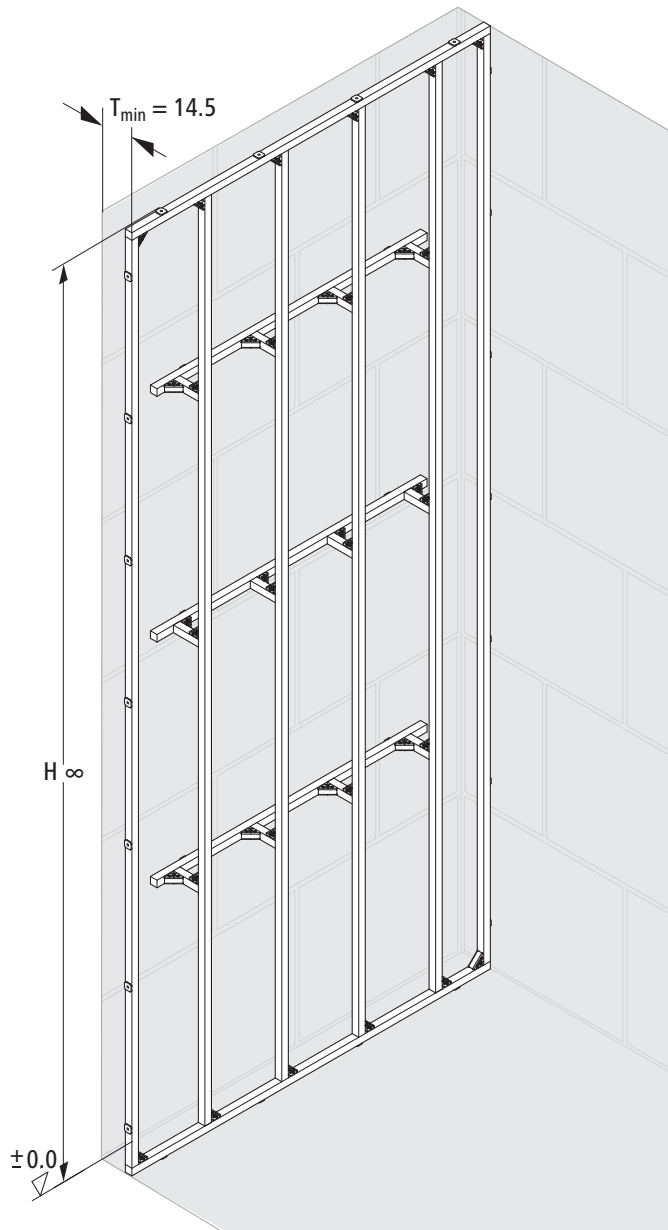
Abb. 1: Optimis-Vorwand, beliebige Höhe
