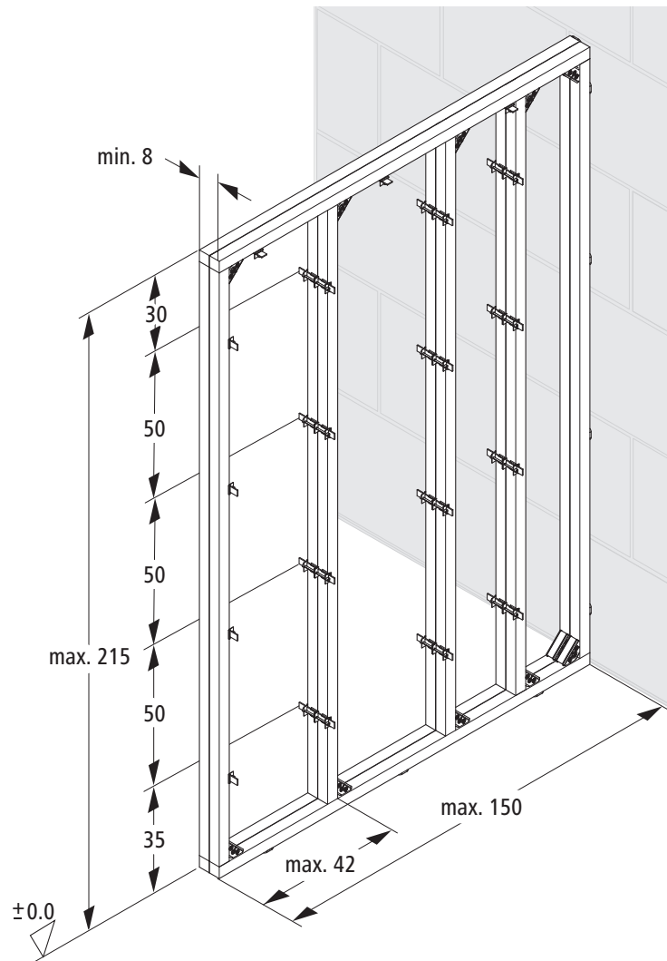
Abb. 17: Montagemasse Flügelwand 8 cm × 150 cm × 215 cm, beplankt, mit Parallelverbinder
