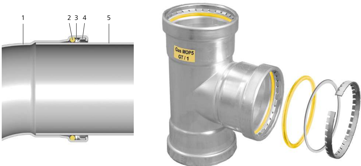
Abb. 2: Optipress-Gaz-XL-Pressverbinding Ø 64, 76.1, 88.9 und 108 mm
