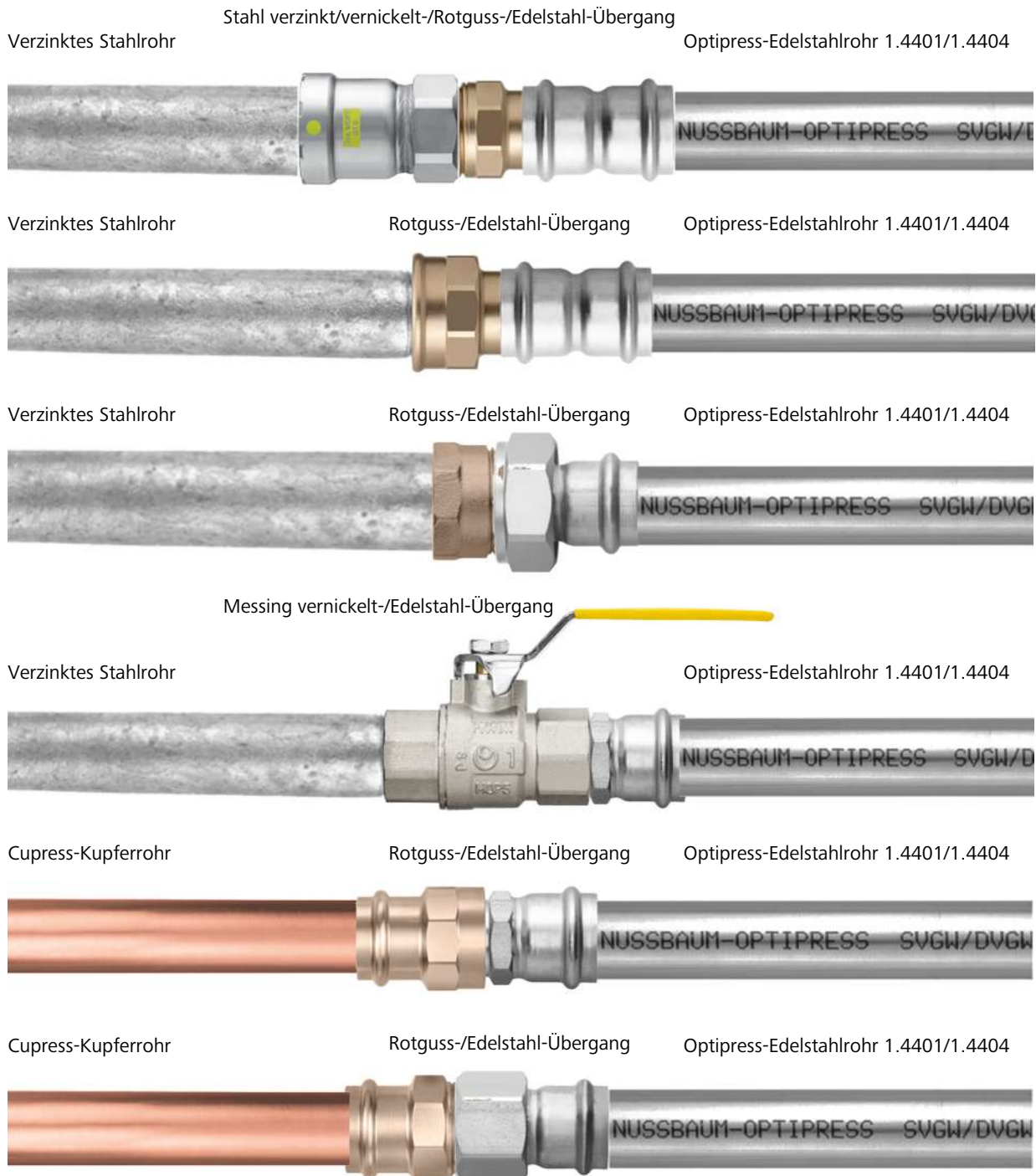
Abb. 3: Zulässige Mischinstallationen mit Optipress-Gaz
