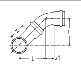
Optipress-Aquaplus-Kombination 80000 / 80004
