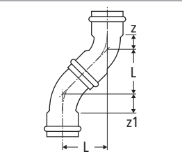
Optipress-Aquaplus-Kombination 80003 / 80004
