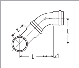
Optipress-Aquaplus-Kombination 80000 / 80004
