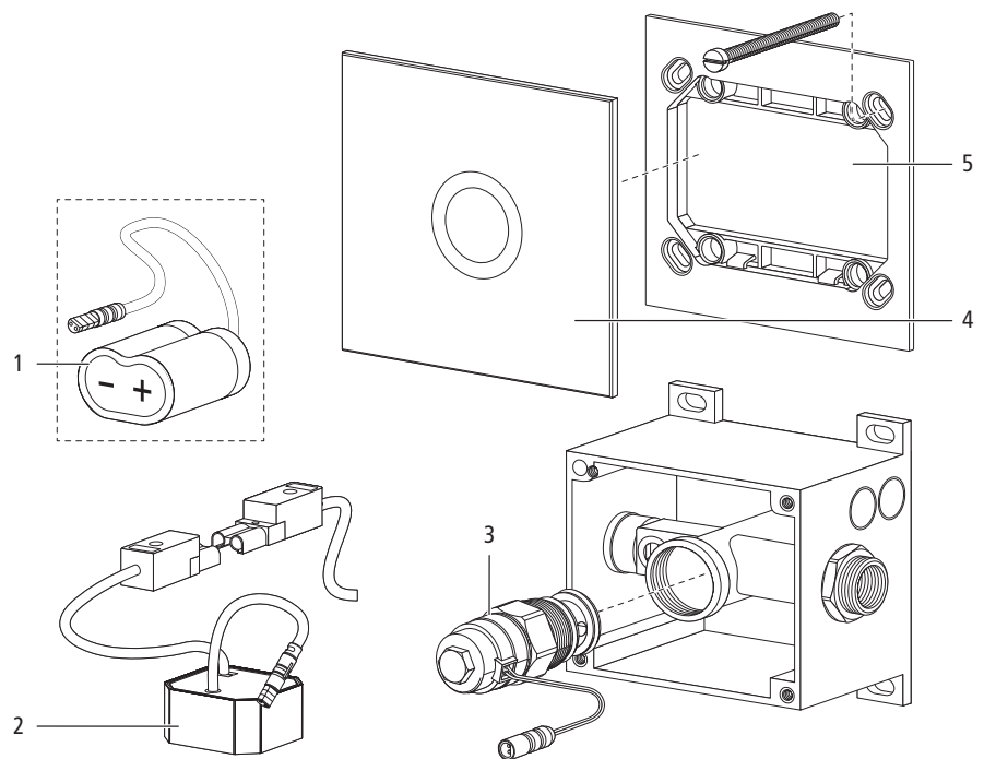
Abb. 3: Ersatzteile Infrarot-Steuerung More 1 (71009)
