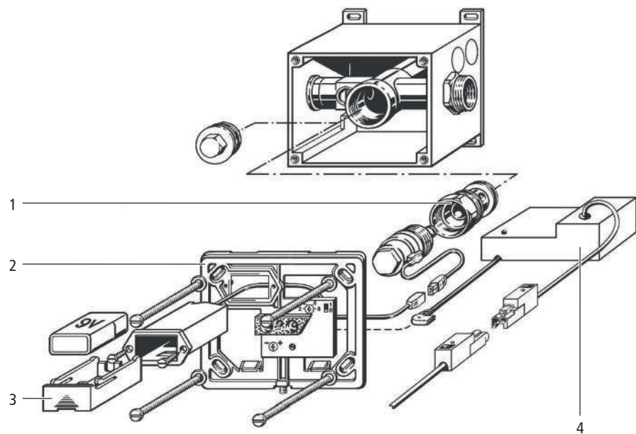
Abb. 2: Ersatzteile Infrarot-Steuerung (71007)
