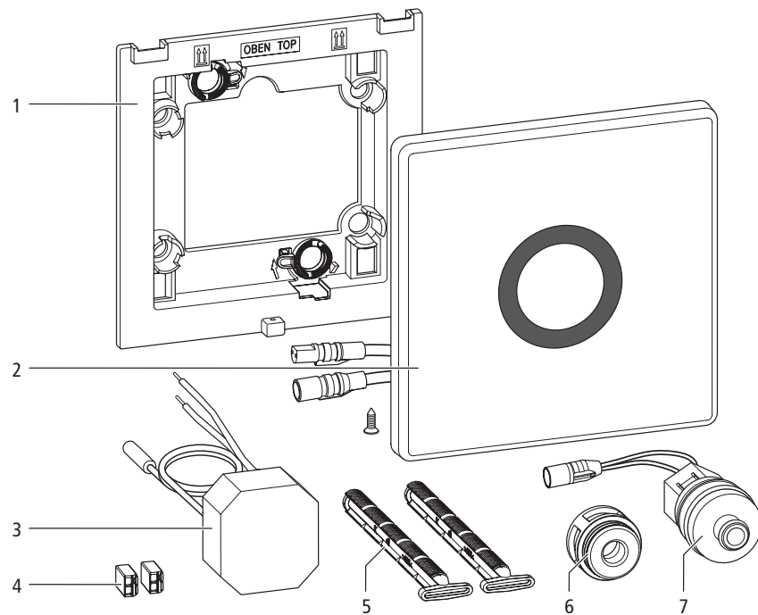
Abb. 4: Ersatzteile Infrarot-Steuerung Public 12 (71286)
