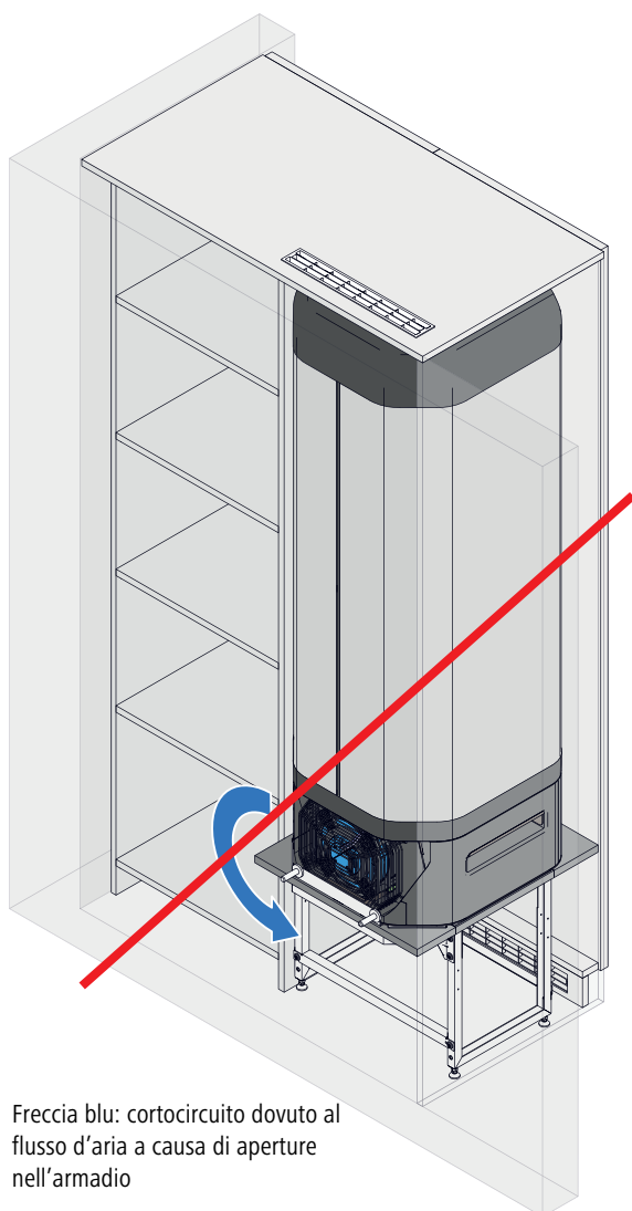
Fig. 4: Misure per evitare cortocircuiti dovuti al flusso d'aria (vista da dietro di una situazione d'installazione)
