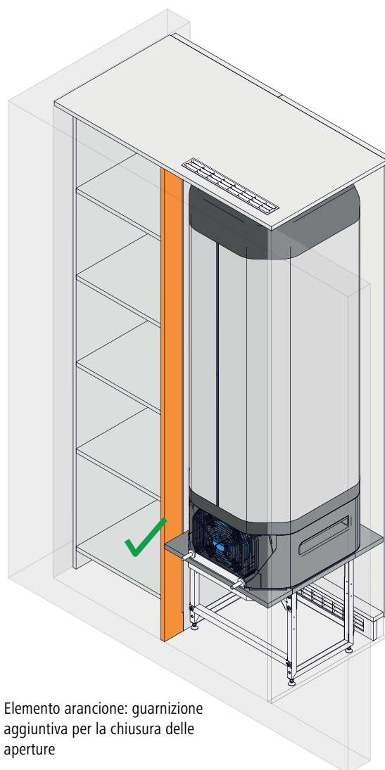
Fig. 4: Misure per evitare cortocircuiti dovuti al flusso d'aria (vista da dietro di una situazione d'installazione)
