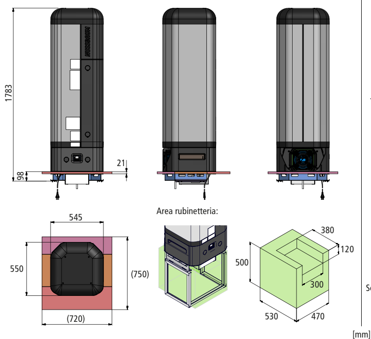
Fig. 2: Condizioni di installazione per apparecchio sostitutivo a incasso, con adattatore per telaio di terzi
