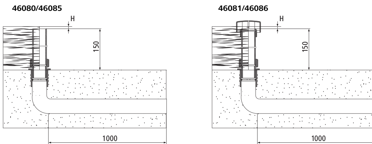
Fig. 1: Determinazione del livello dell'acqua (nelle immagini ad es. 150 mm)
