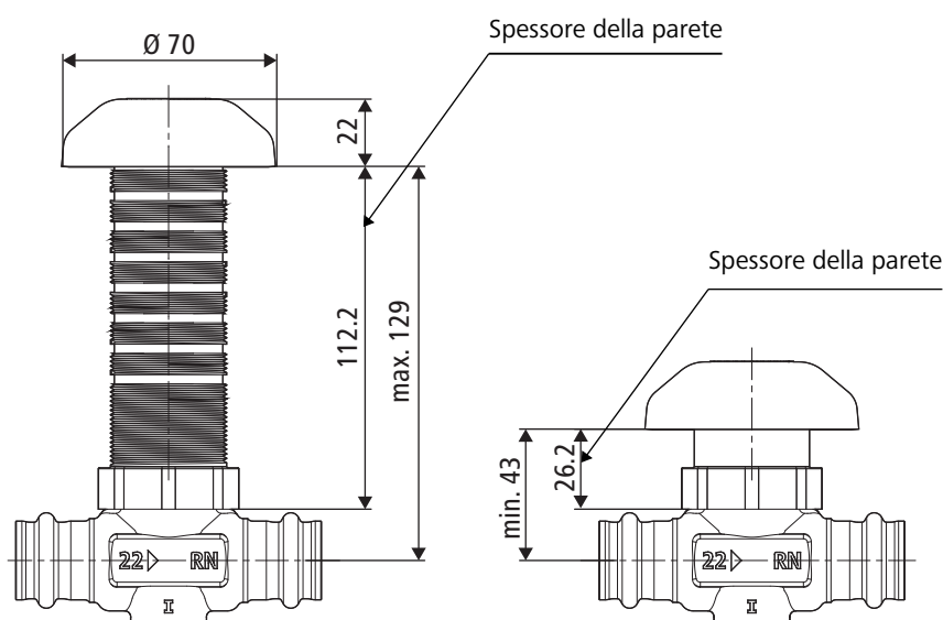
Fig. 1: Situazione d'installazione parete cantiere
