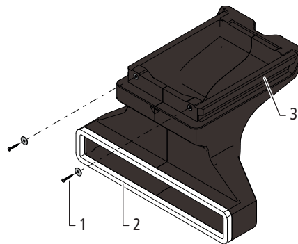
Abb. 7: Luftführung Zuluft 68014
