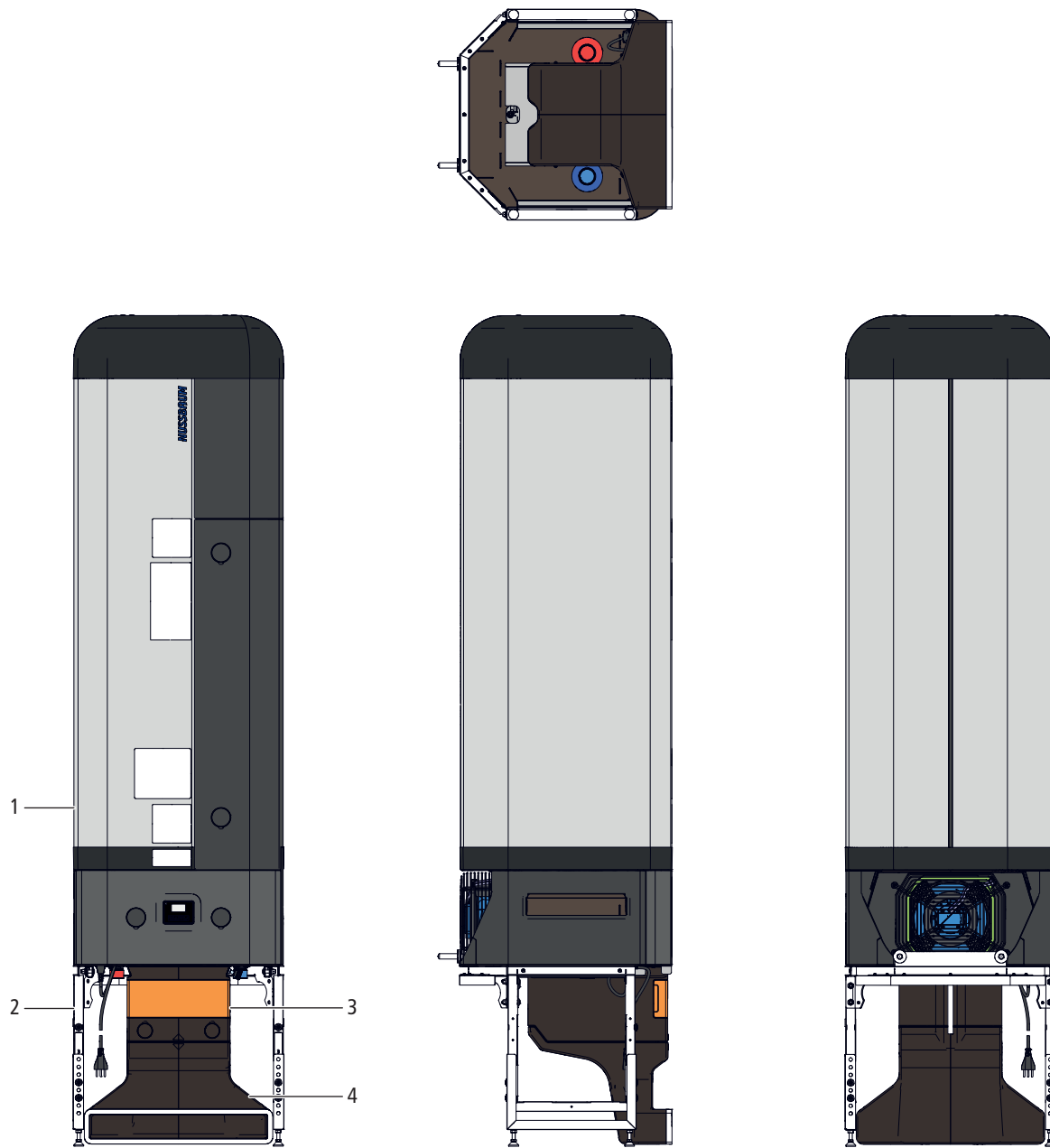
Abb. 4: Gerät 68010.21
