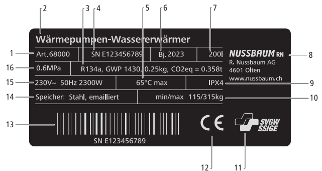
Abb. 8: Typenschild
