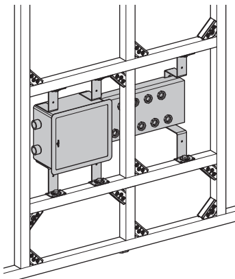
Unterputz-Armaturenbox 70110 (horizontal)
