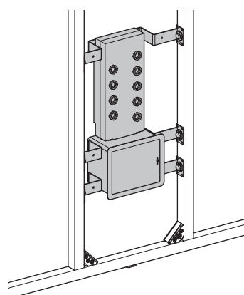
Unterputz-Armaturenbox 70112 (vertikal)
