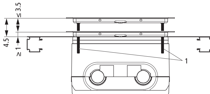
1 Schraube M5 × 50
