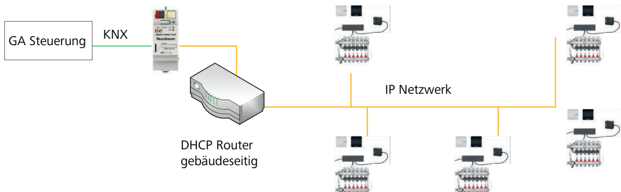
Abb. 6: Anschlussschema Therm-Control-KNX-Modul
