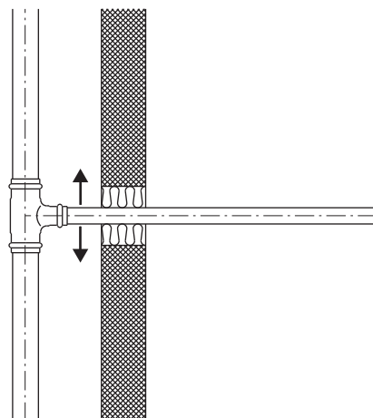
Abb. 3: Spielraum für die vertikale Verschiebung des Abgangs der Etagenleitung
