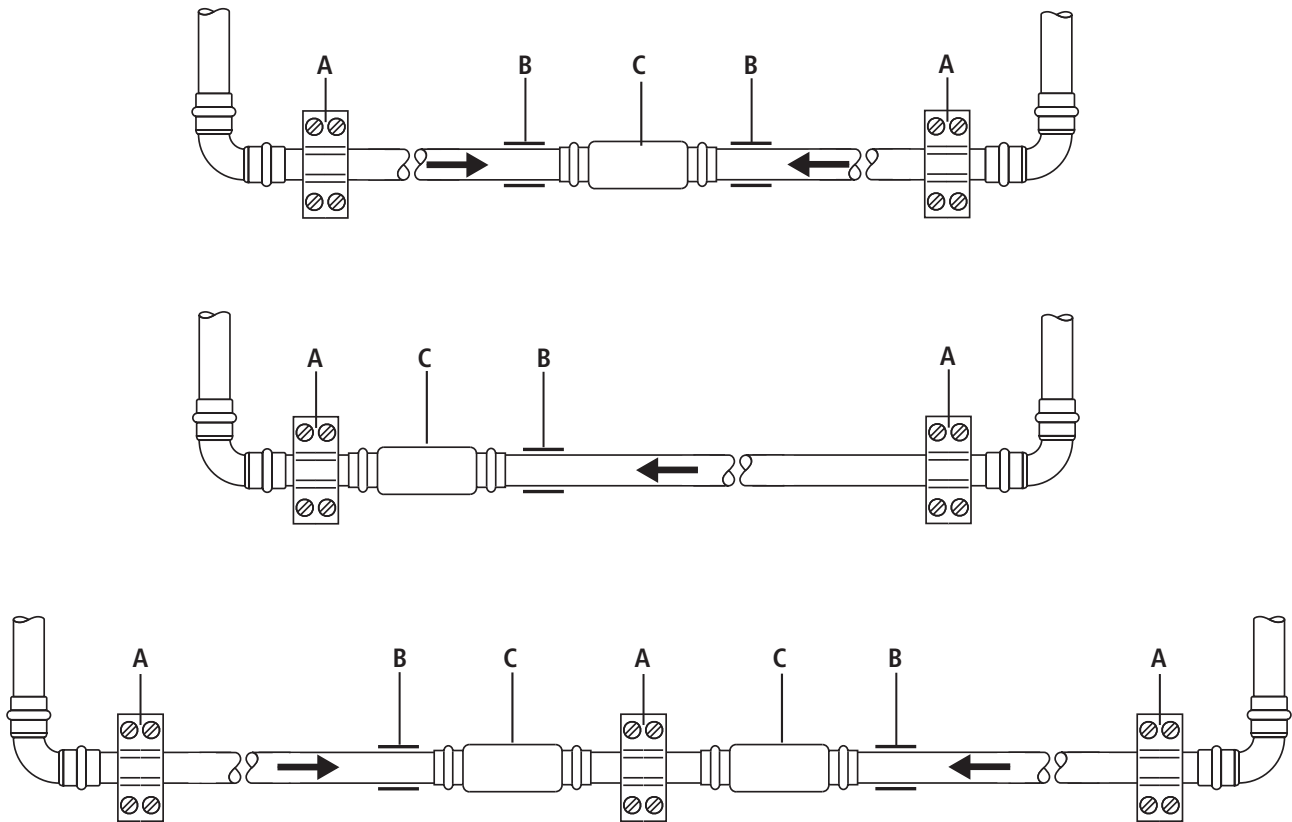
Abb. 1: Montagebeispiele Längenkompensator
