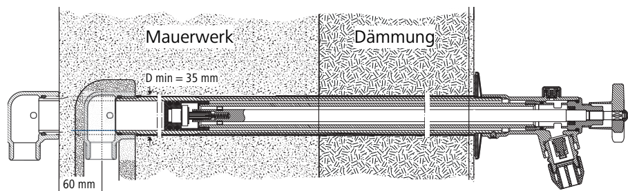
Abb. 1: Montagesituation Aussendämmung
