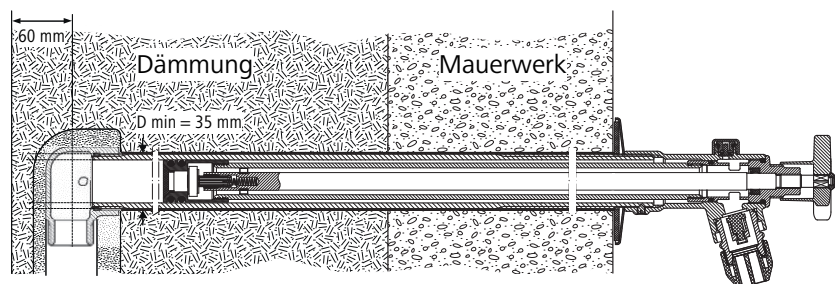
Abb. 2: Montagesituation Innendämmung
