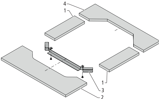
Fig. 6: Guarnizione camera 68021, con staffa di supporto
