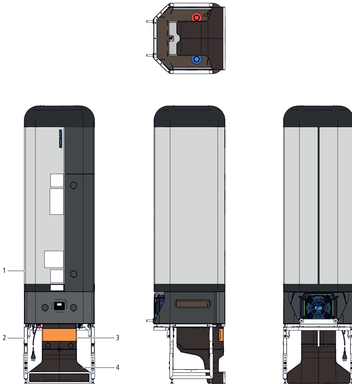
Fig. 4: Apparecchio 68010.21
