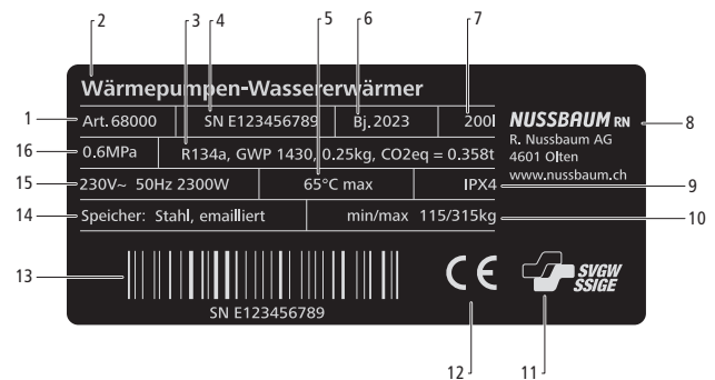
Fig. 8: Targhetta
