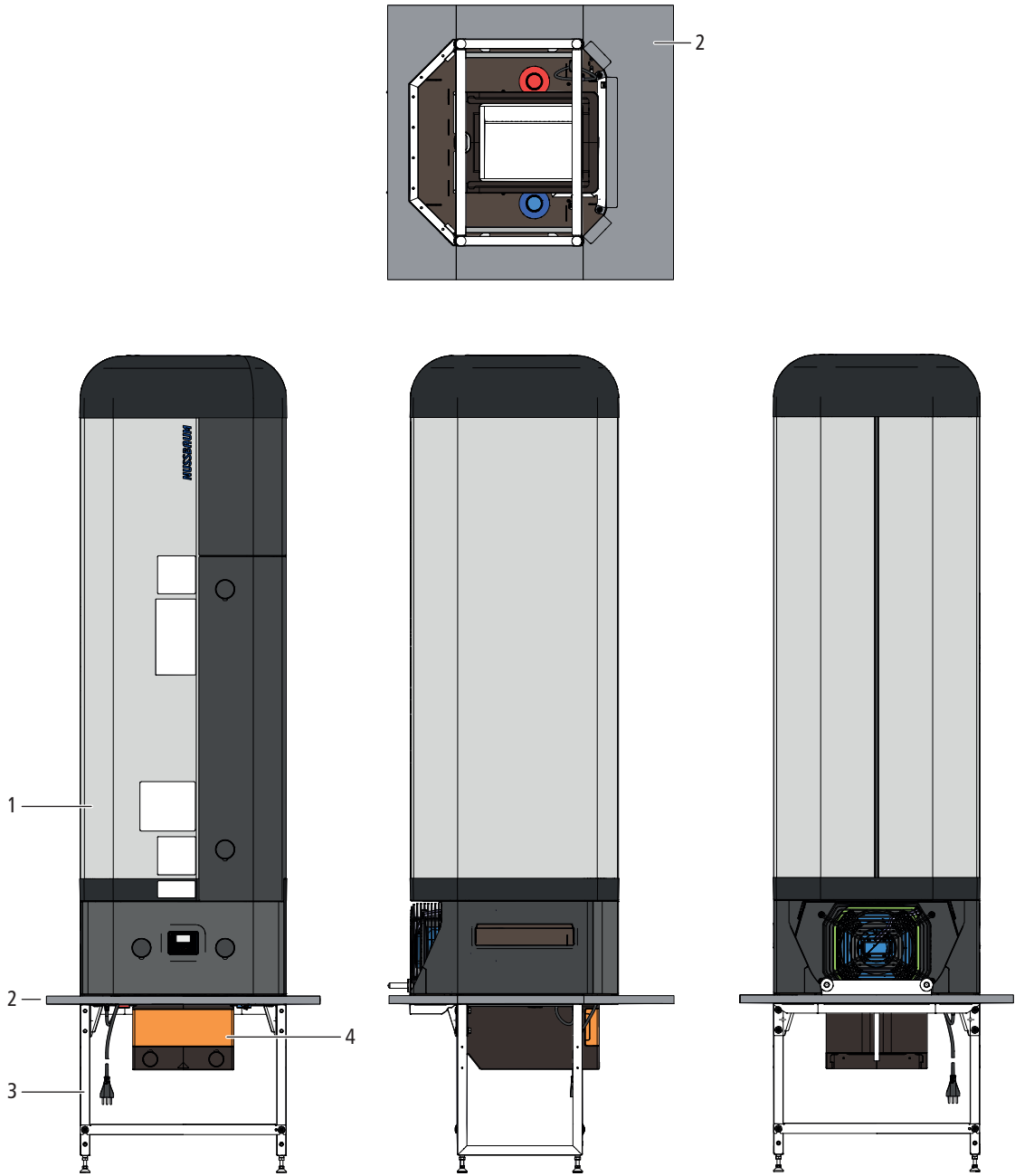
Fig. 3: Apparecchio 68020.21
