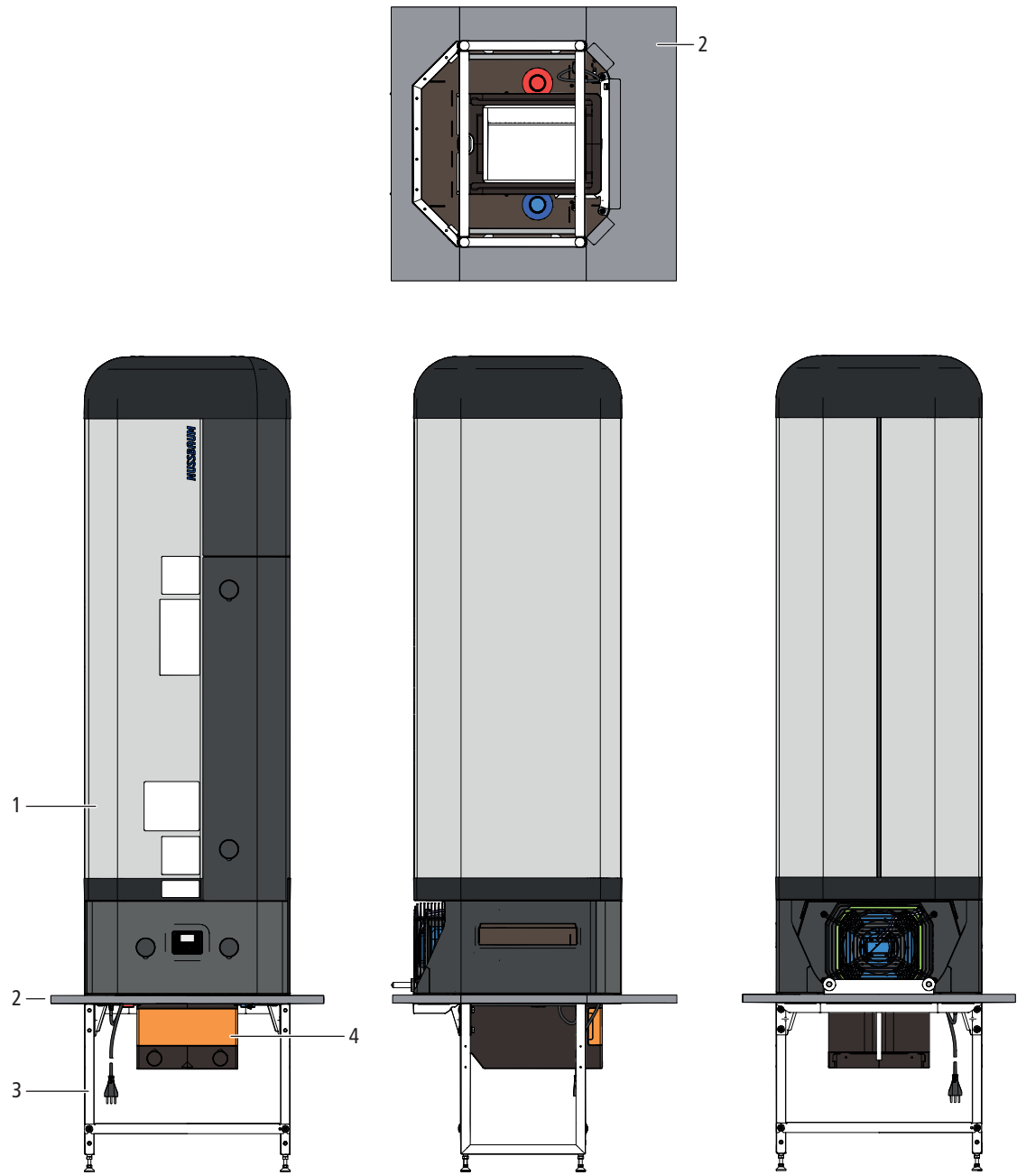
Fig. 3: Apparecchio 68020.21
