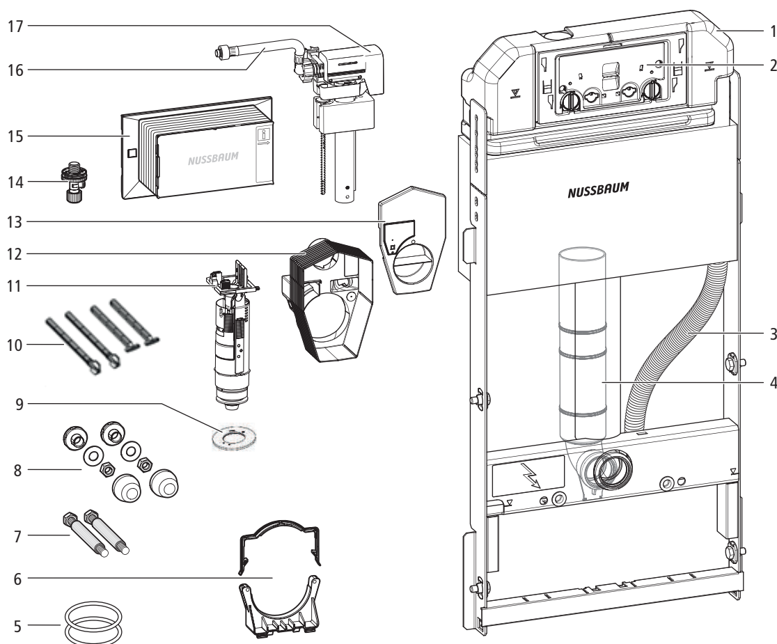
Fig. 1: Struttura del modulo WC Optimis-Tec 71200
