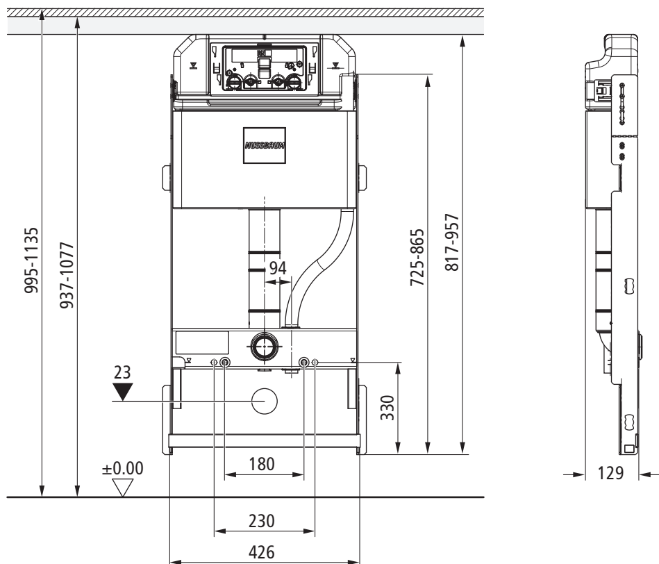
Fig. 2: Misure d'installazione modulo WC Optimis-Tec
