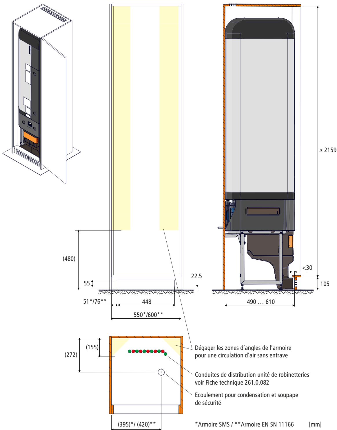
Fig. 14: Schéma de pose armoire SMS / SN EN 1116:2018
