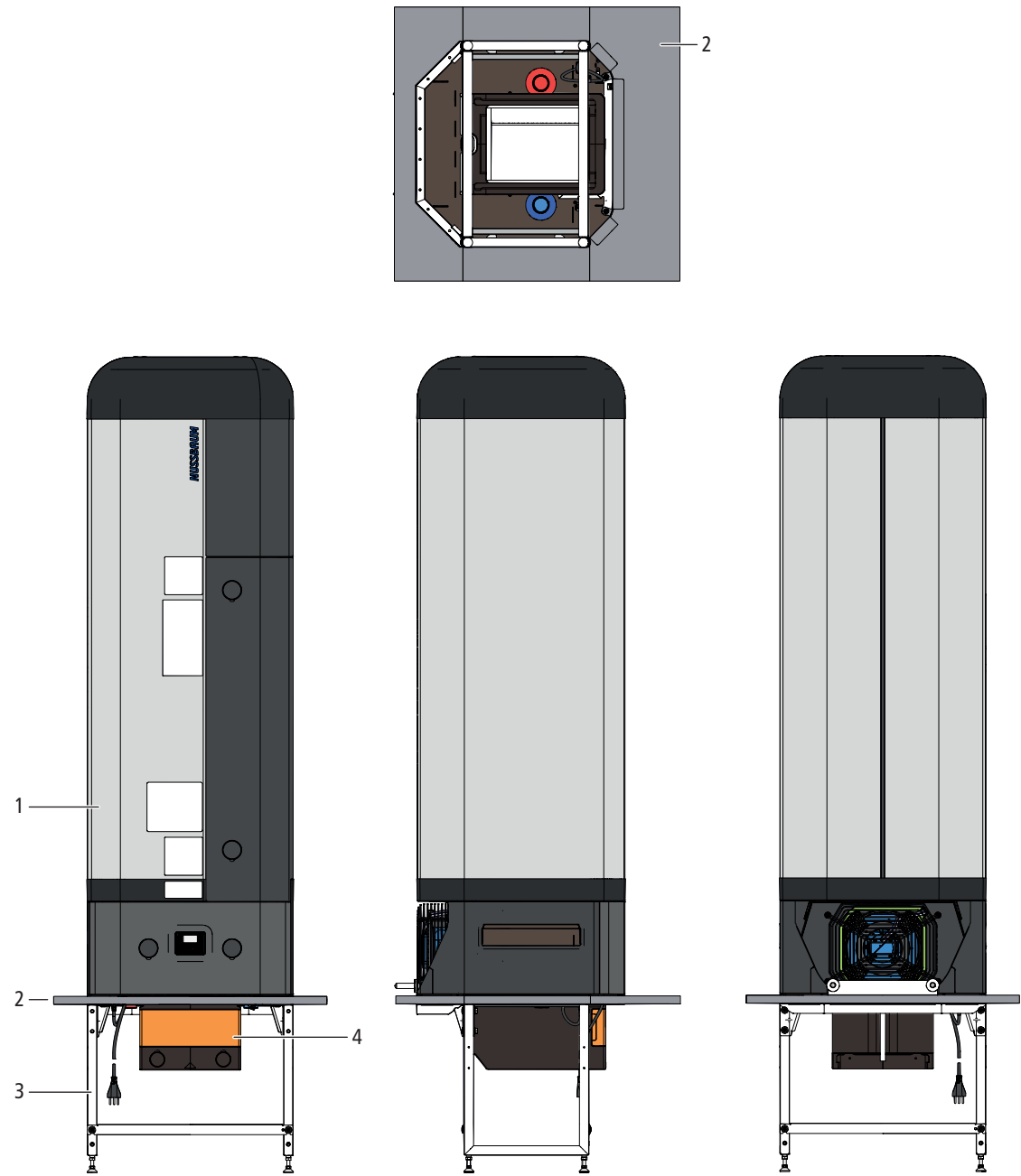
Fig. 3: Appareil 68020.21
