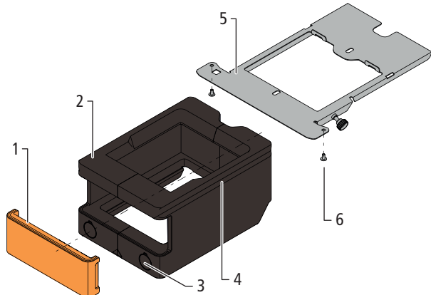
Fig. 4: Corps du filtre à air (sans filtre à air) 68013 et rail de guidage 68967
