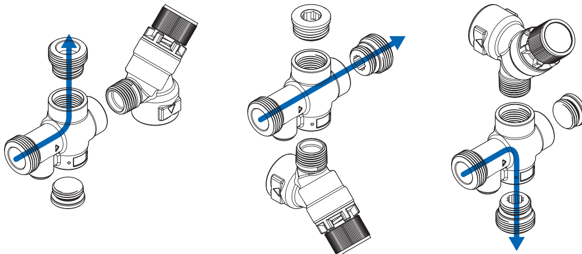
Fig. 1: Un écoulement direct vers le chauffe-eau est assuré dans n'importe quelle position
