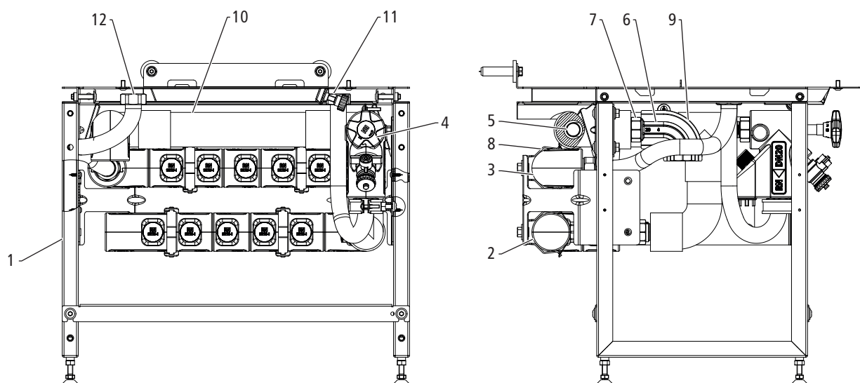
Fig. 3: Garniture de robinetterie 68080.25
