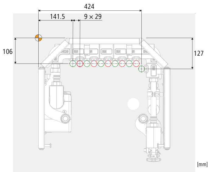
Fig. 5: Schéma de pose des conduites de distribution dans la partie inférieure de l'armoire
