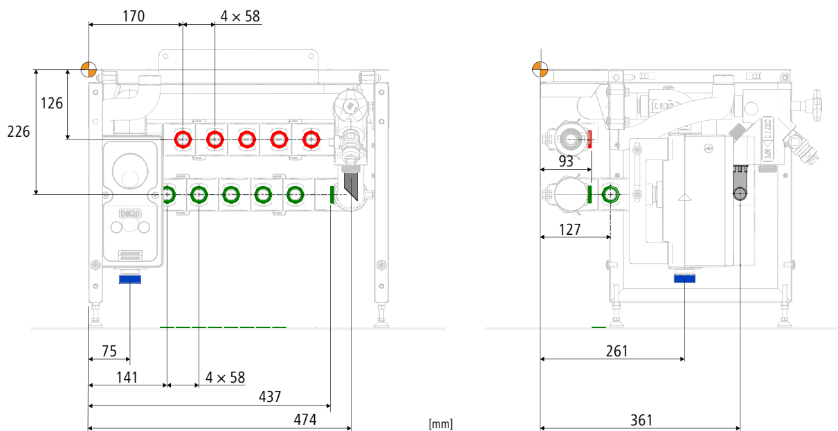
Fig. 4: Bleu: accouplement rapide alimentation eau froide DN20; vert/rouge: conduites de distribution PWC/PWH pièces intermédiaires enfichables; gris: tubulure d'écoulement
