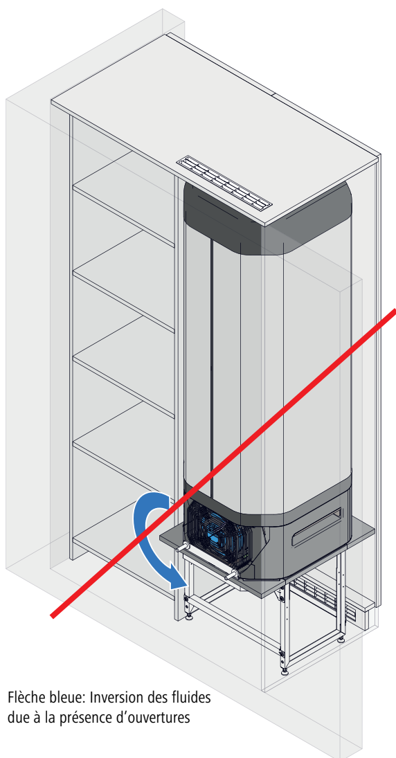
Fig. 4: Empêcher une inversion des fluides (vue arrière d'un montage en particulier)
