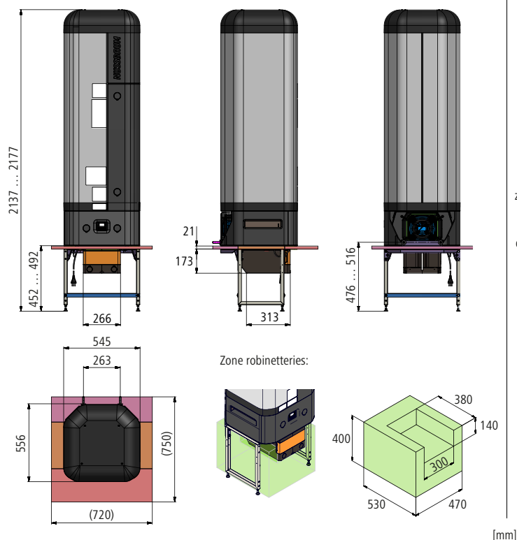
Fig. 2: Conditions de pose pour appareil de remplacement, avec soubassement Nussbaum
