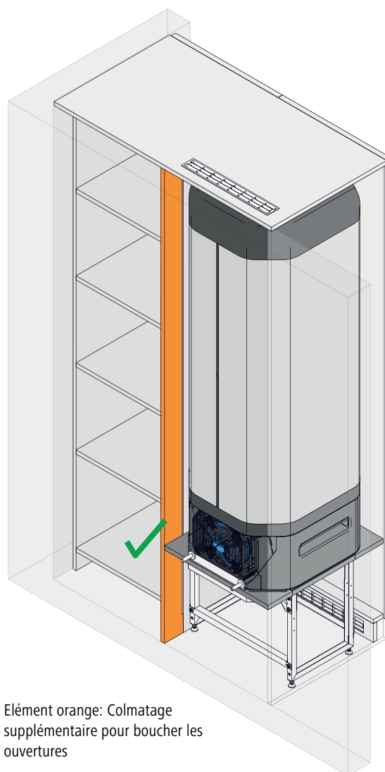
Fig. 4: Empêcher une inversion des fluides (vue arrière d'un montage en particulier)
