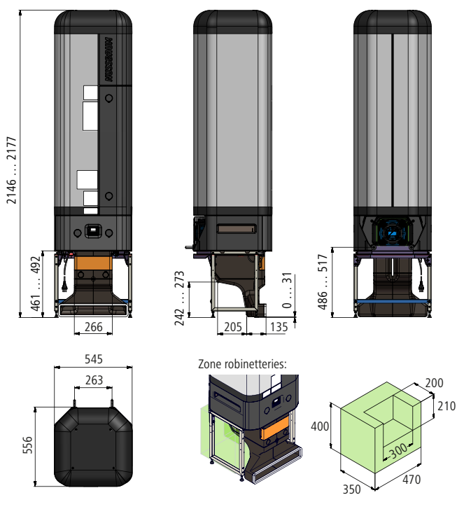
Fig. 3: Conditions de pose pour les appareils dans les armoires SMS / SN EN 1116:2018
