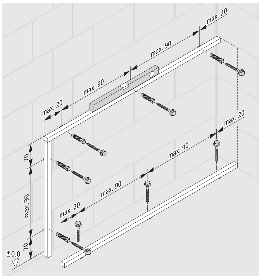
Fig. 8: Misure di montaggio per preparare a mezza altezza, fissaggio alla parete posteriore (costruzione massiccia)
