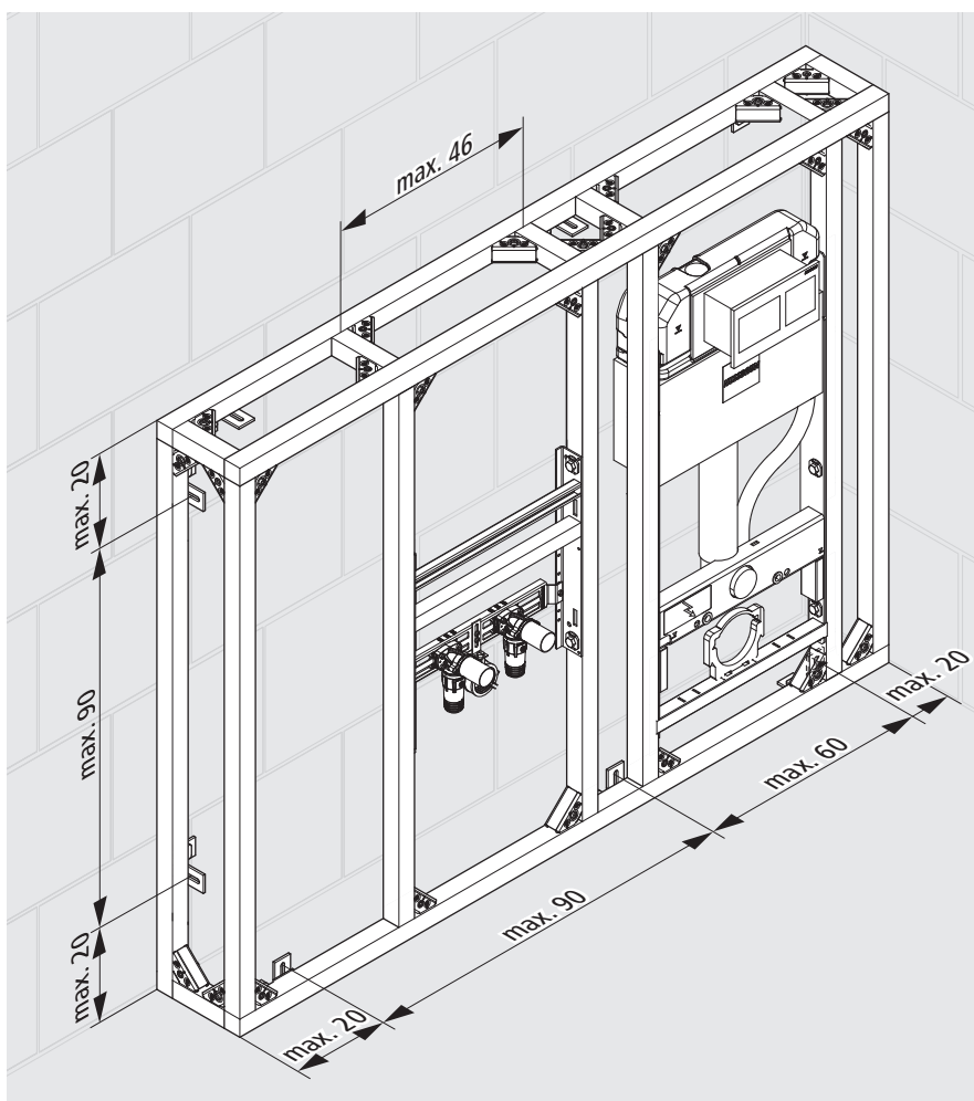
Fig. 21: Misure di montaggio per preparare a mezza altezza.
