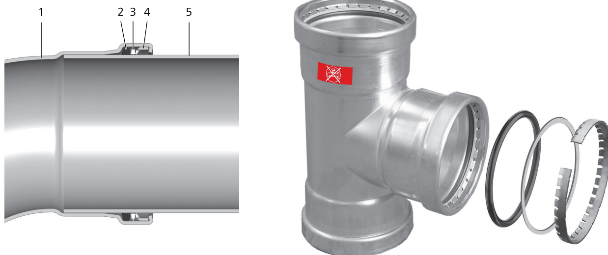
Fig. 2: Raccordo a pressione Optipress-Therm XL Ø 64, 76.1, 88.9 e 108 mm
