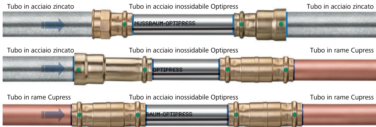
Fig. 4: Installazioni miste consentite con Optipress-Industry
