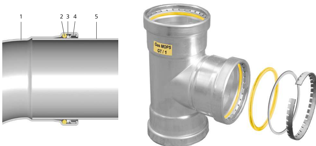
Fig. 2: Raccordo a pressare Optipress-Gaz XL Ø 64.0, 76.1, 88.9 e 108.0 mm
