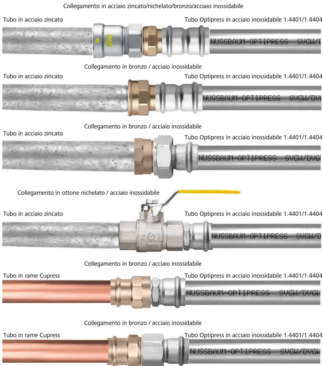
Fig. 3: Installazioni miste consentite con Optipress-Gaz
