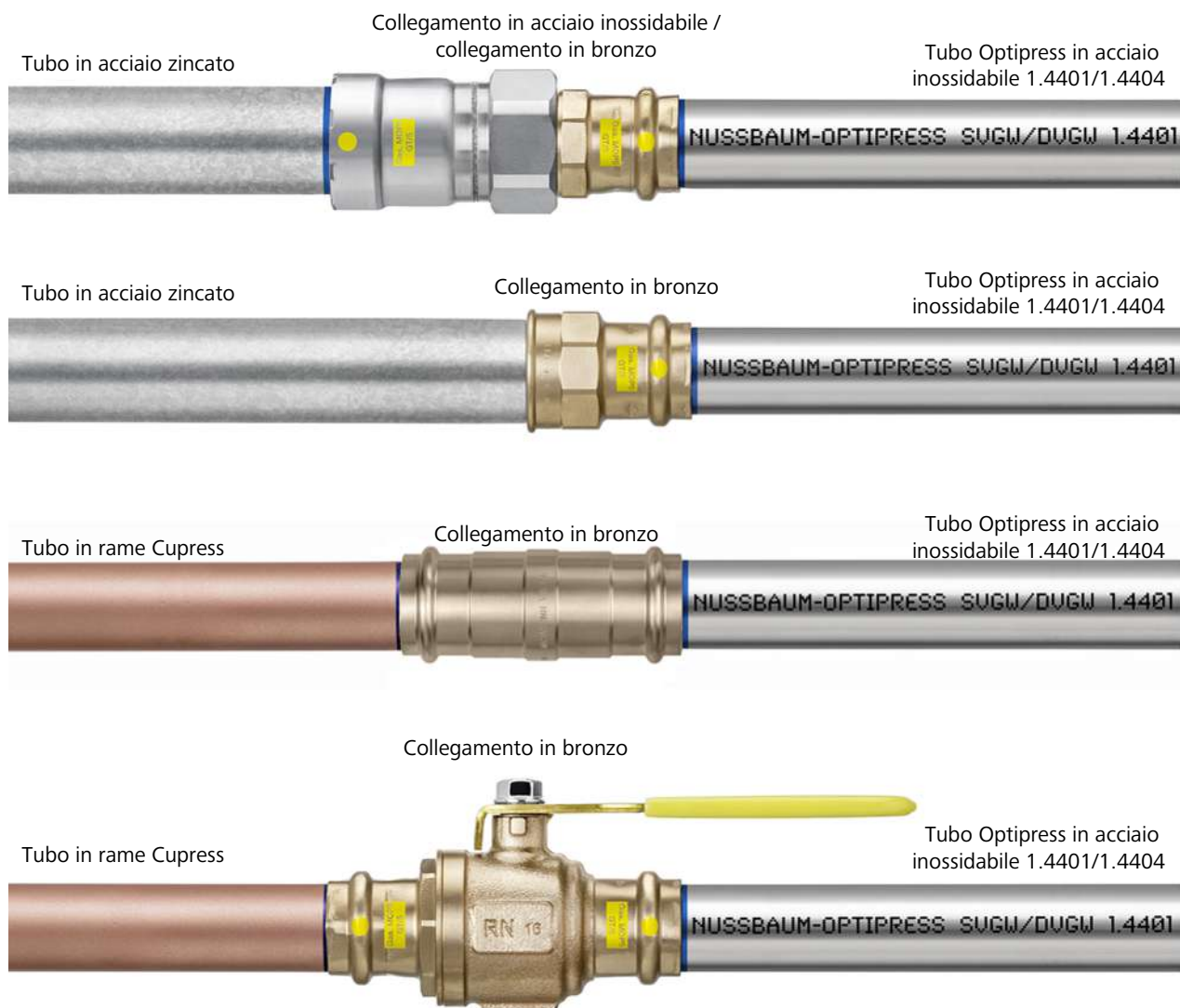
Fig. 3: Installazioni miste consentite con Optipress-Gaz
