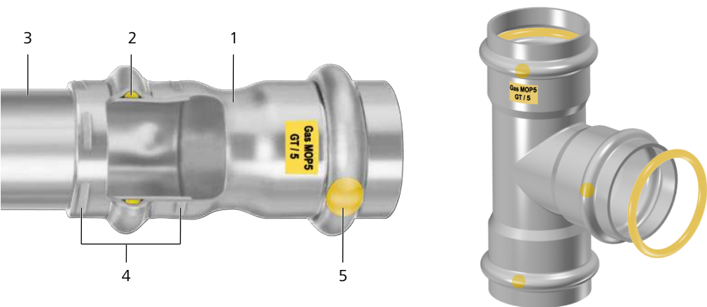
Fig. 1: Raccordo a pressare Optipress-Gaz Ø 15-54 mm
