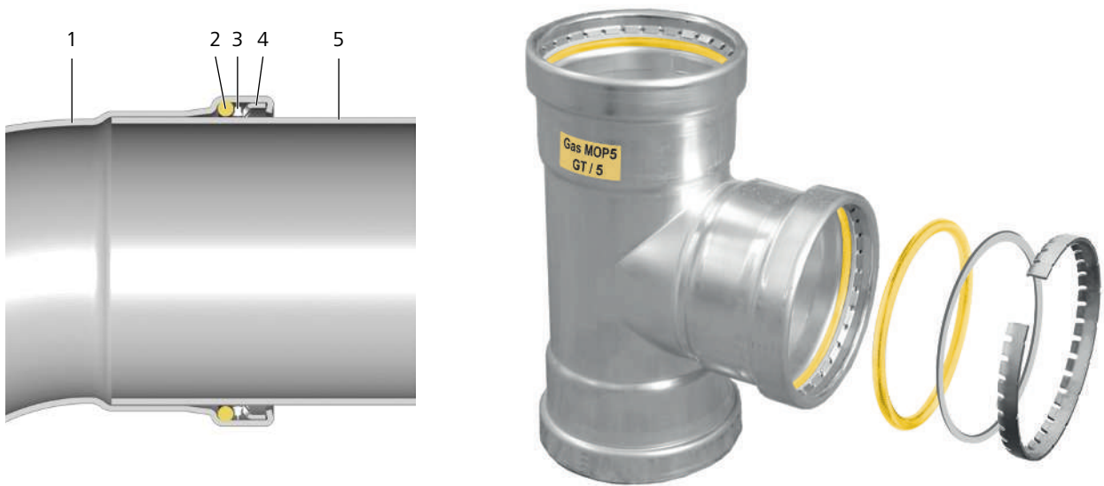
Fig. 2: Raccordo a pressione Optipress-Gaz XL Ø 64,0, 76,1, 88,9 e 108,0 mm
