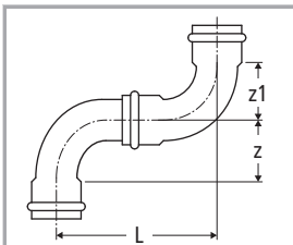
Combinazione Optipress-Gaz 88000 / 88001
